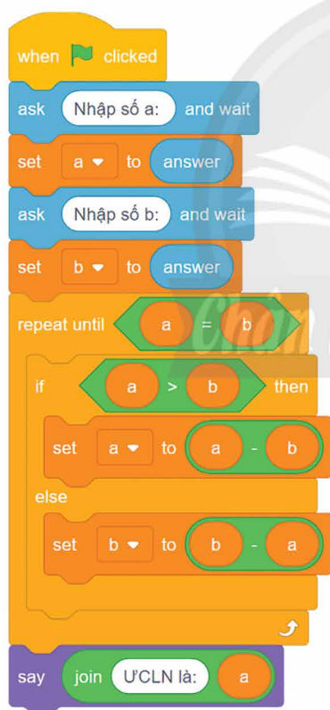
Hình 2a. Chương trình Scratch tìm ƯCLN của hai số nguyên dương a, b
