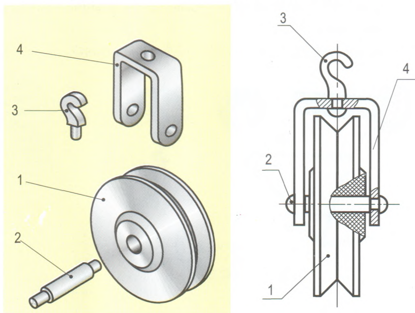
Hình 24.3. Cấu tạo ròng rọc
