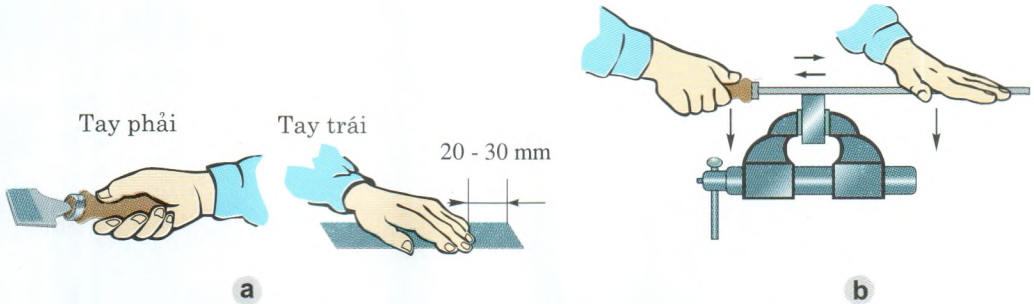
Hình 22.2. Cách cầm dũa và thao tác dũa
