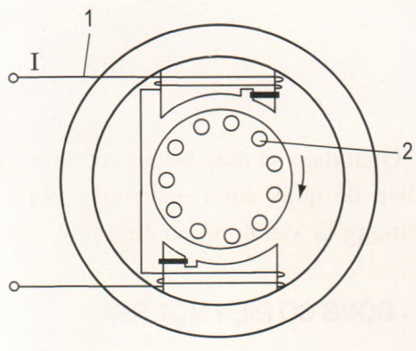
Hình 44.3. Sơ đồ nguyên lí
