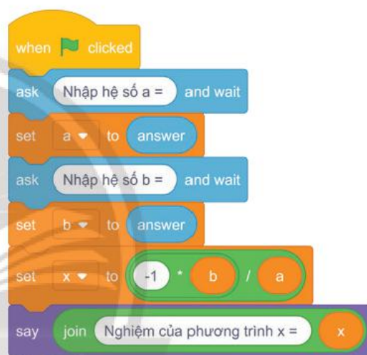
Hình 4. Chương trình tìm nghiệm phương trình ax + b = 0
