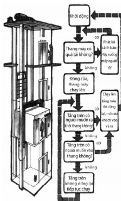
Sơ đồ vận hành của thang máy
