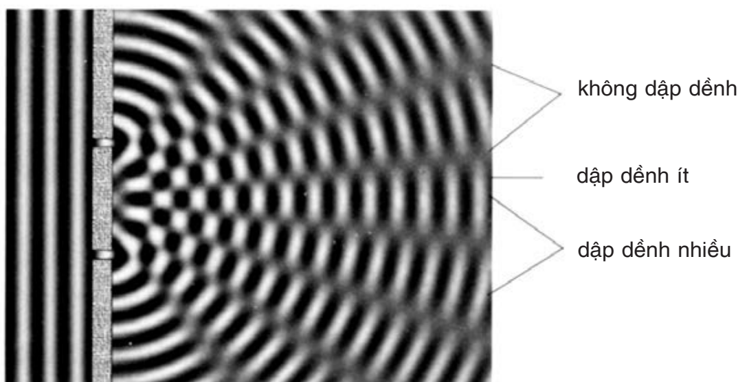
Hình 4.7 Các sóng nước tròn ló ra từ hai khe chồng lên nhau tạo ra sóng tổng hợp được tăng cường ở một số nơi và yếu đi ở một số nơi khác.
