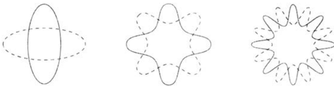
Hình 6.2 Các vòng dây trong lý thuyết dây cũng có thể dao động theo các mode cộng hưởng, tương tự như các dây đàn violon, trong đó một số nguyên các đỉnh và hõm sóng được đặt vừa khít dọc theo chiều dài của chúng.
