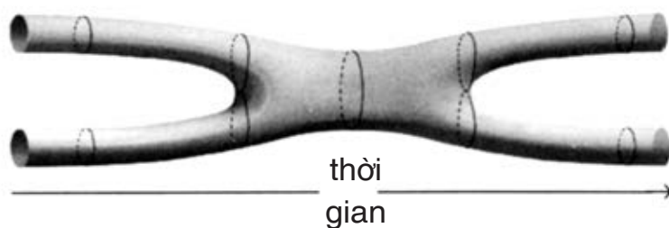
Hình 12.3 Các dây tương tác bằng cách nhập vào và tách ra.
