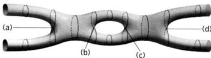
Hình 12.4 Sự náo nhiệt lượng tử có thể sinh ra cặp dây/phản dây (b) rồi hủy nhau (c) làm cho tương tác trở nên phức tạp hơn.
