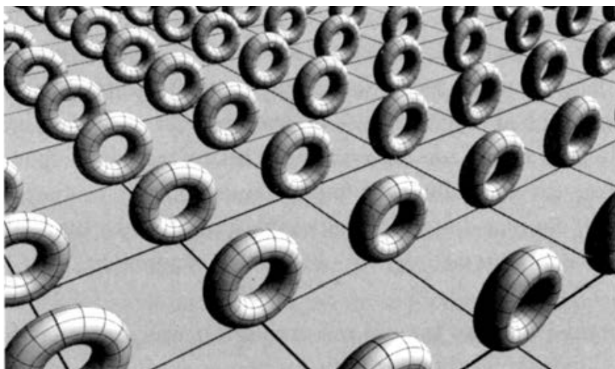
Hình 8.8 Hai chiều phụ cuộn thành một mặt hình xuyên.
