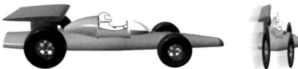
Hình 2.4 Một vật chuyển động bị co ngắn lại theo phương chuyển động.
