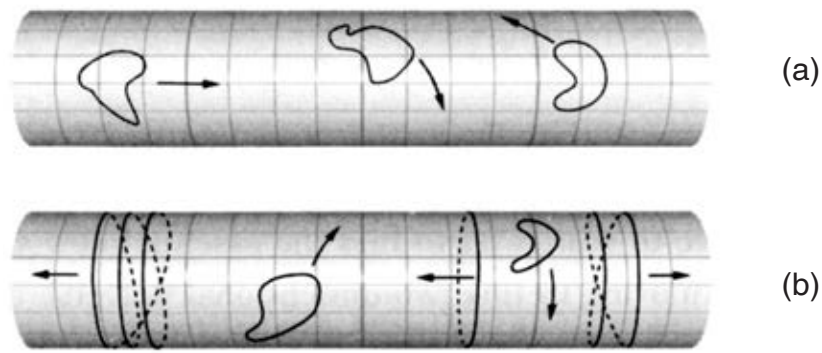
Hình 10.3 Các dây có thể chuyển động trên mặt ống nước theo hai cách: theo cấu hình không xoắn và cấu hình xoắn quanh ống.
