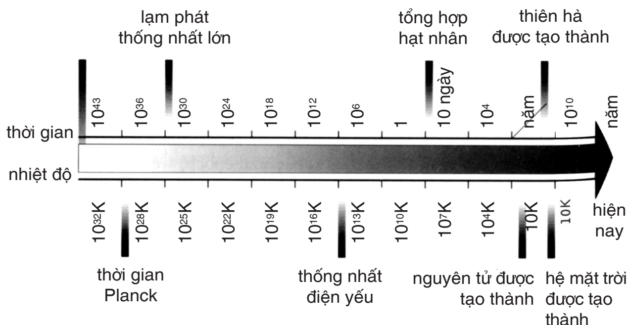
Hình 14.1 Đường thẳng thời gian ghi lại những thời điểm then chốt trong lịch sử của Vũ trụ.
