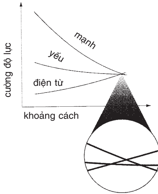
Hình 7.2 Sự hoàn thiện tính toán các cường độ lực cho thấy, nếu không có siêu đối xứng, chúng chỉ gần chứ không hoàn toàn hội tụ với nhau.
