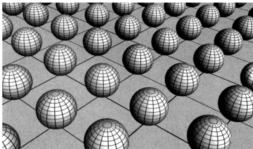
Hình 8.7 Hai chiều phụ cuộn thành một mặt cầu.
