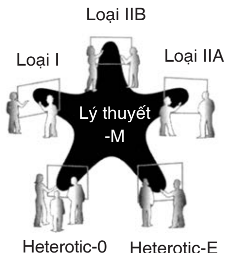
Hình 12.2 Kết quả của cuộc cách mạng siêu dây lần thứ hai đã chứng tỏ rằng tất cả năm lý thuyết dây thực sự là một bộ phận của một khuôn khổ thống nhất duy nhất mà người ta tạm gọi là lý thuyết-M.
