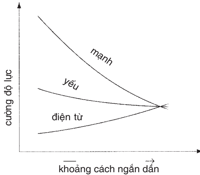
Hình 7.1 Cường độ của ba lực phi hấp dẫn ở những thang khoảng cách ngắn dần, hay tương đương thế, trong những quá trình có năng lượng cao dần.
