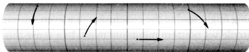
Hình 10.2 Các hạt điểm chuyển động trên mặt ống nước.
