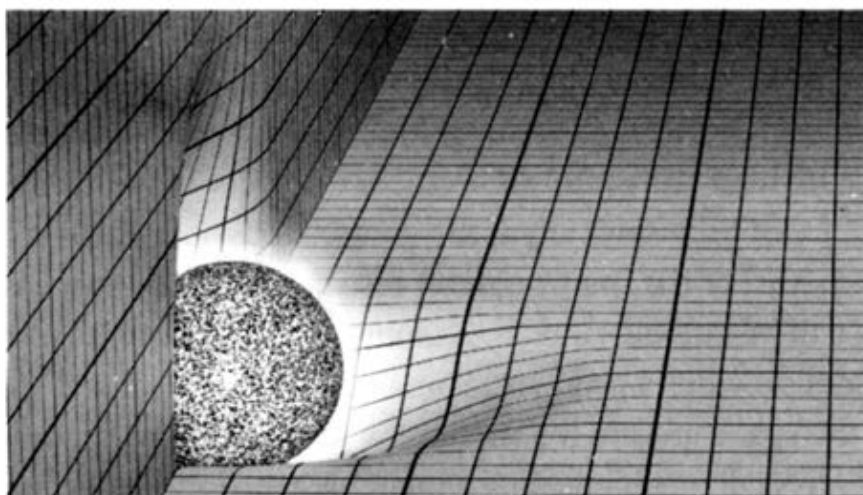
Hình 3.6. Một mẫu về sự cong của không gian ba chiều xung quanh Mặt trời
