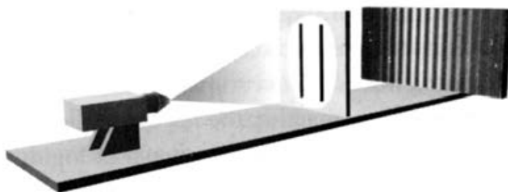
Hình 4.8 Nếu ánh sáng là sóng, thì khi cả hai khe đều mở, sẽ có sự giao thoa giữa các sóng tới từ hai khe.
