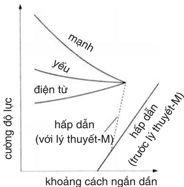
Hình 14.2 Bên trong lý thuyết-M, cường độ của tất cả bốn lực có thể hòa nhập một cách tự nhiên.
