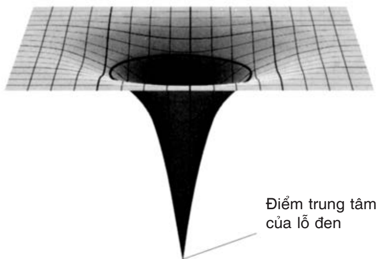
Hình 3.7. Lỗ đen làm cong cấu trúc không-thời xung quanh mạnh tới mức bất kỳ vật nào rơi vào bên trong “chân trời sự kiện” của nó - được minh họa bằng vòng tròn đen trên hình - đều không thoát khỏi móng vuốt hấp dẫn của nó. Chưa ai biết chính xác điều gì sẽ xảy ra ở điểm bên trong sâu nhất của lỗ đen.
