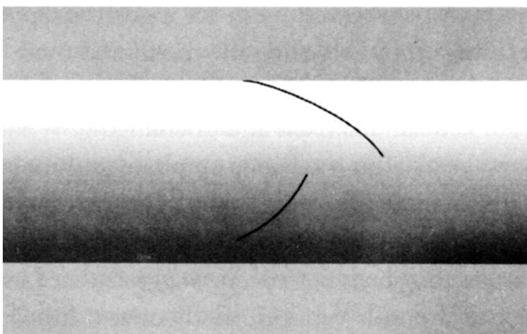
Hình 8.5. Một cư dân Xứ sở Thăng có thể nhìn thấy trực tiếp nội tạng của một cư dân khác khi xứ sở này giãn nở thành vũ trụ ống nước.
