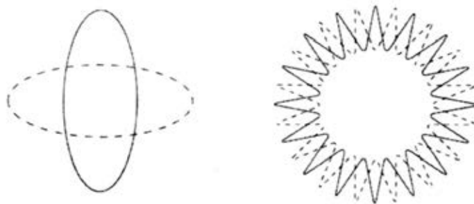
Hình 6.3 Mode dao động mãnh liệt sẽ có năng lượng lớn hơn mode dao động lò dờ.
