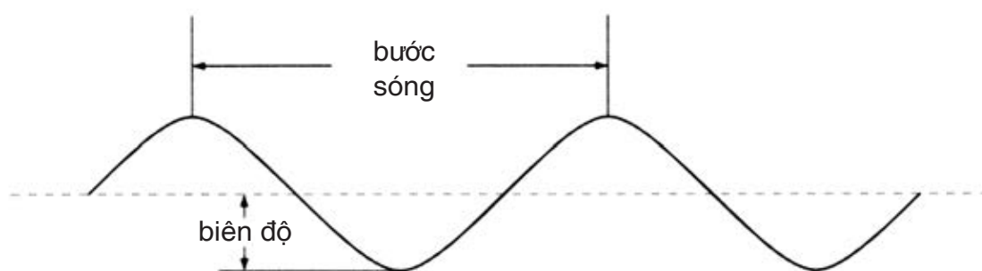
Hình 4.2 Bước sóng là khoảng cách giữa hai đỉnh hoặc hai hõm sóng liên tiếp. Biên độ là độ cao hoặc độ sâu cực đại của sóng.
