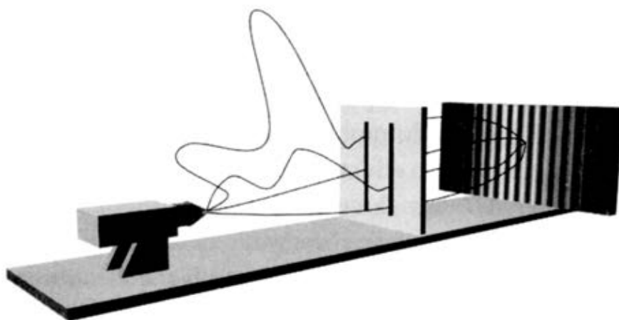
Hình 4.10 Theo cách trình bày cơ học lượng tử của Feynman, cần phải xem rằng các hạt đi từ điểm này tới điểm khác theo mọi quỹ đạo khả dĩ. Trên hình có vẽ một ít trong số vô hạn các quỹ đạo khả dĩ từ nguồn tới màn huỳnh quang. Chú ý rằng electron này thực sự đi qua cả hai khe.
