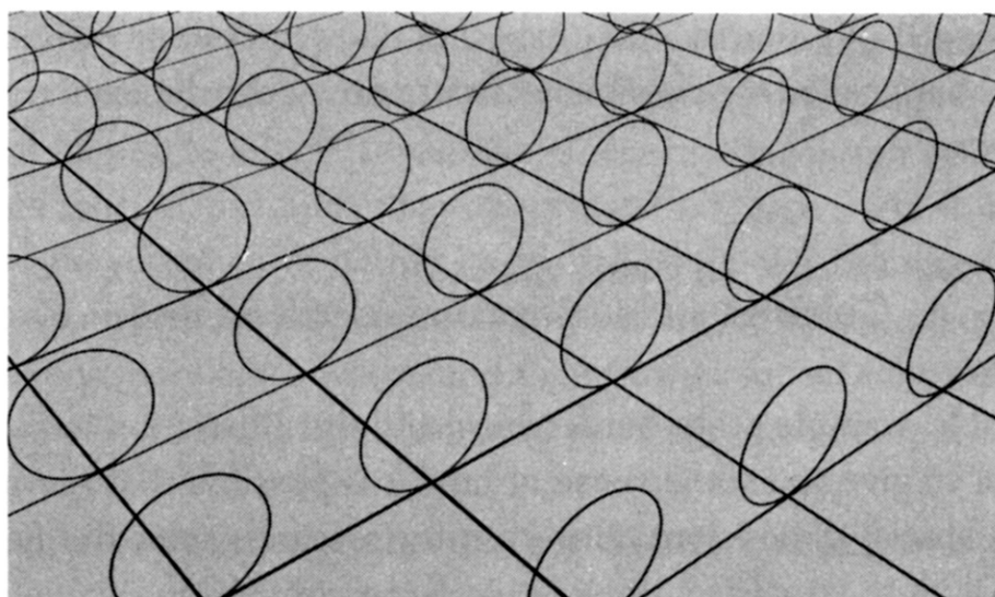
Hình 8.4 Những đường kẻ ô biểu diễn các chiều lớn quen thuộc trong đời sống hằng ngày của chúng ta, trong khi đó các vòng tròn biểu diễn chiều mới, chiều nhỏ và bị cuộn tròn lại. Giống như những vòng sợi len xếp chặt tạo nên lớp xốp của một tấm thảm, những vòng tròn này tồn tại ở mỗi điểm trong các chiều lớn quen thuộc, nhưng để dễ nhìn ta chỉ vẽ chúng tại giao điểm của các đường kẻ ô.
