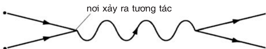
Hình 6.6 Trong lý thuyết trường lượng tử, một hạt và phản hạt của nó có thể tức thời hủy nhau và tạo ra một photon. Sau đó, photon này có thể sinh ra một hạt khác và một phản hạt đi theo những quỹ đạo khác.
