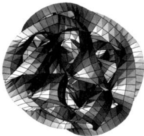
Hình 8.9 Một ví dụ về không gian Calabi-Yau
