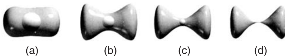
Hình 11.3 Một mặt cầu trong không gian Calabi-Yau co lại thành một điểm, làm đứt cấu trúc không gian. Hình này và các hình tiếp sau đã được đơn giản hóa bằng cách chỉ vẽ phần có liên quan của không gian Calabi-Yau có chứa mặt cầu.
