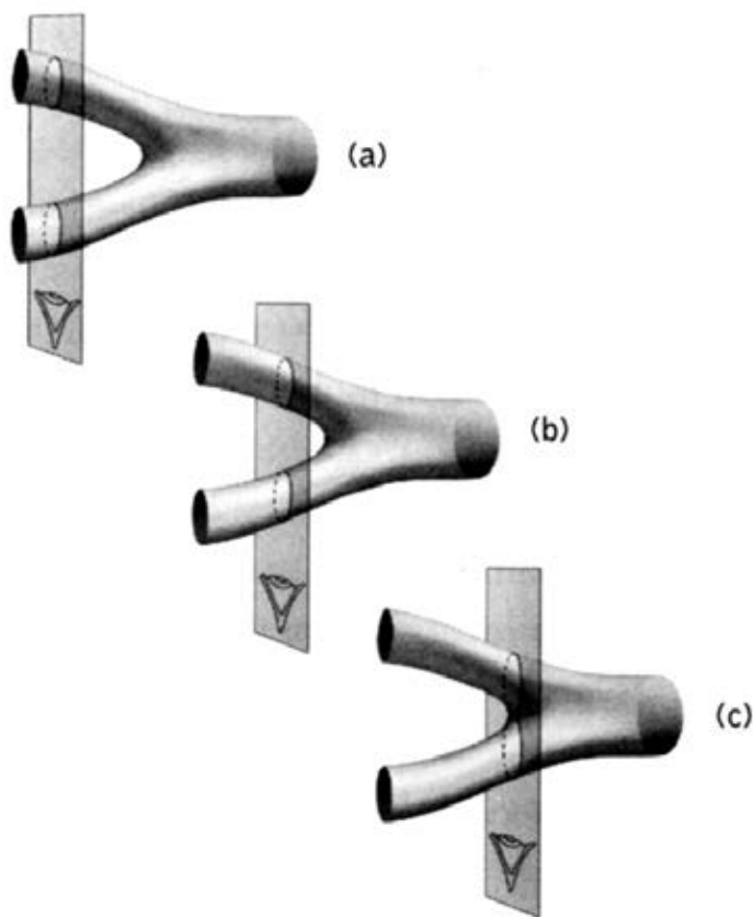
Hình 6.8 Hai dây chuyển động tới gặp nhau ở ba thời điểm theo quan điểm của George. Trong (a) và (b) các dây đang tiến lại gần nhau và ở (c) chúng lần đầu tiên chạm vào nhau, theo quan điểm của George.
