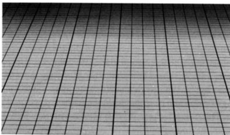
Hình 3.3 Biểu diễn một không gian phẳng
