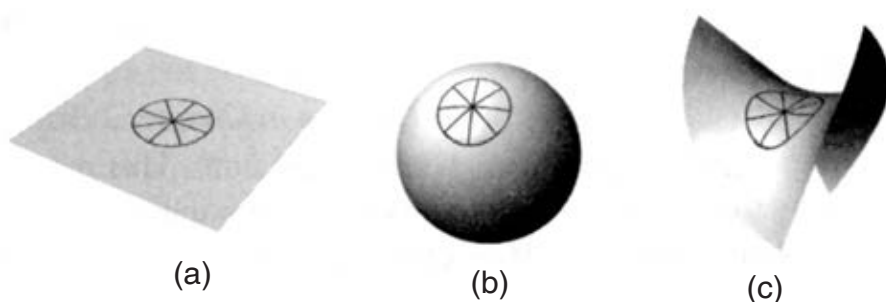
Hình 3.2 Vòng tròn được vẽ trên mặt cầu (b) có chu vi nhỏ hơn vòng tròn vẽ trên mặt phẳng (a), trong khi đó vòng tròn vẽ trên mặt hình yên ngựa (c) lại có chu vi lớn hơn ngay cả khi chúng có bán kính như nhau.
