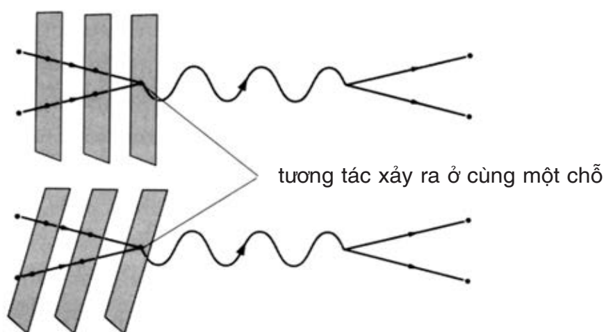
Hình 6.11 Những người quan sát chuyển động đối với nhau nhất trí về nơi và thời điểm diễn ra tương tác của hai hạt điểm.
