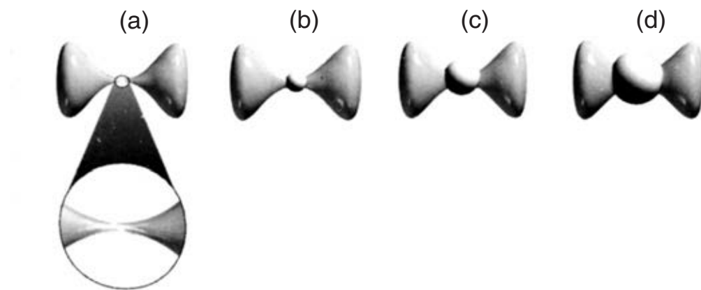
Hình 11.4 Một không gian Calabi-Yau bị thắt được mở ra và một mặt cầu mọc ra, lớn dần lên làm trơn bề mặt của không gian đó.
