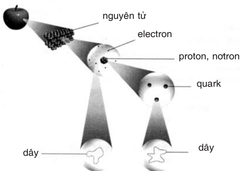
Hình 1.1. Vật chất được cấu tạo từ các nguyên tử, rồi các nguyên tử lại được tạo thành từ các quark và electron. Theo lý thuyết dây, tất cả các hạt đó lại được tạo thành từ các dây dao động.
