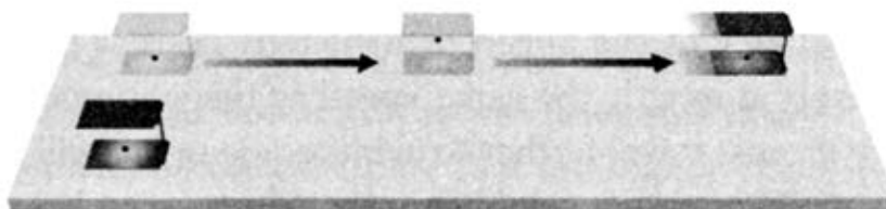
Hình 2.2 Chiếc đồng hồ photon ở phía trước đứng yên, trong khi đó chiếc đồng hồ thứ hai chuyển động thẳng đều.
