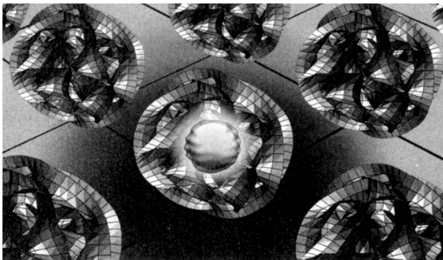
Hình 13.4 Khi một brane bao quanh một mặt cầu ở trong các chiều bị cuộn lại, nó nhìn giống như một lỗ đen trong các chiều rộng lớn quen thuộc.
