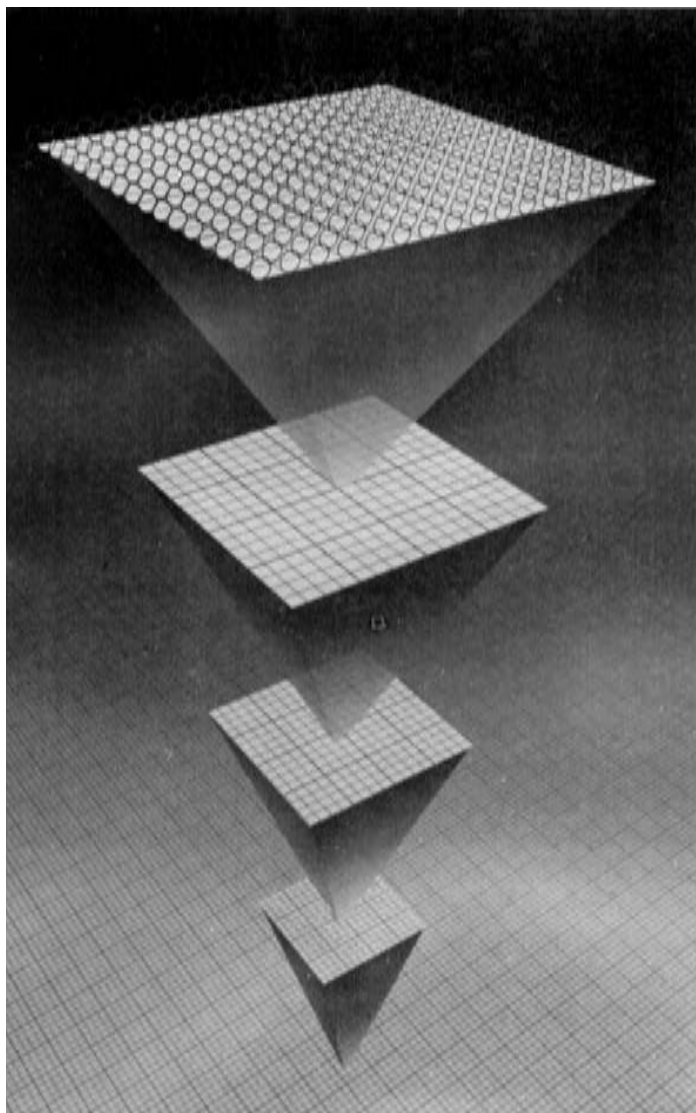
Hình 8.3 Giống như Hình 5.1, mỗi một mức tiếp sau biểu diễn hình phóng đại lớn hơn của cấu trúc không gian ở mức trước. Vũ trụ của chúng ta có thể có các chiều phụ, như được thấy ở mức phóng đại thứ tư, nếu như chúng được cuộn lại trong một không gian nhỏ tới mức cho tới nay chúng ta vẫn chưa phát hiện được.
