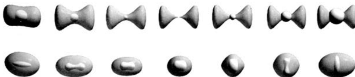
Hình 11.5 Một dịch chuyển lật xé rách không gian (hàng trên) và cũng dãy tiến hóa đó nhưng trong không gian ảnh (hàng dưới).
