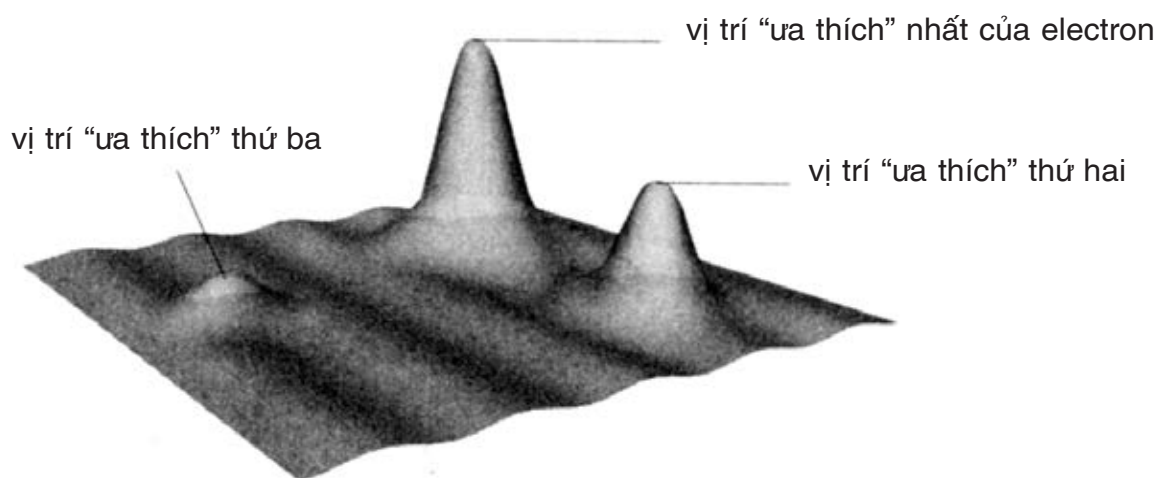
Hình 4.9 Sóng gắn với electron là lớn nhất ở những nơi thường hay tìm thấy nó nhất và sóng dần dần nhỏ hơn ở những nơi ít tìm thấy nó hơn.
