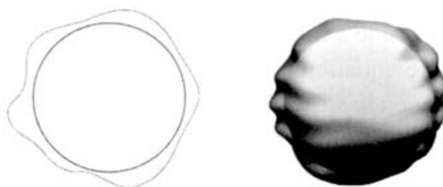
Hình 13.1 Dây có thể bao quanh một mẫu một chiều của cấu trúc không-thời gian bị cuộn lại; còn một màng hai chiều có thể bao quanh một mẫu hai chiều.
