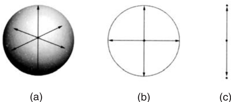
Hình 13.2 Các mặt cầu với số chiều dễ hình dung: số chiều của (a) là hai; của (b) là một và của (c) là không.
