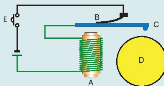
Hình 20.4 Sơ đồ cấu tạo chuông điện
