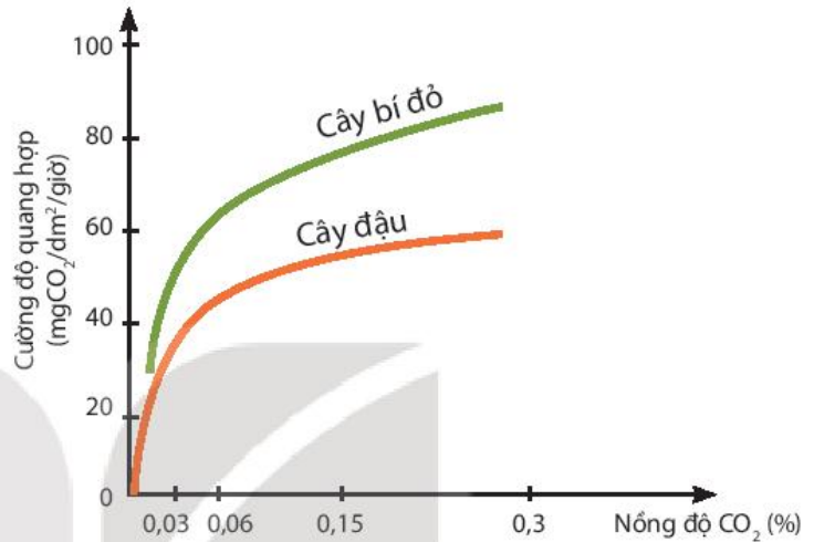
Hình 23.2 Đồ thị thể hiện ảnh hưởng của nồng độ khí \text{CO}_2 ngoài môi trường đến quang hợp ở cây bí đỏ và cây đậu*
