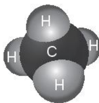
b) Methane
