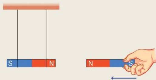
Hình 18.4 Thí nghiệm tìm hiểu tương tác giữa hai nam châm
