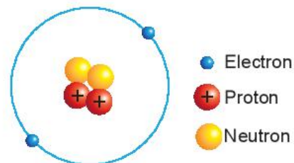
Hình 2.4 Mô hình nguyên tử helium
