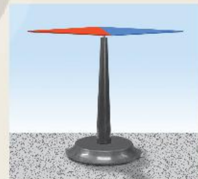
Hình 18.3 Kim nam châm
