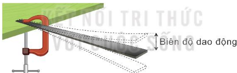
Hình 13.1 Thí nghiệm quan sát thước dao động
