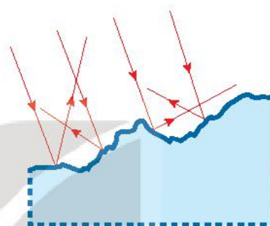
Hình 16.4 Phản xạ khuếch tán
