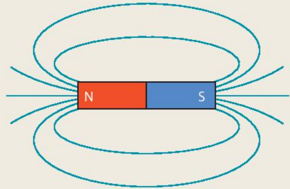
Hình 19.3 Mô tả đường sức từ
