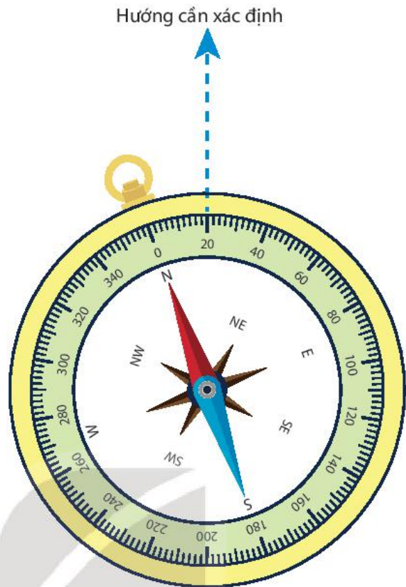
Hình 19.9 Cách sử dụng la bàn
