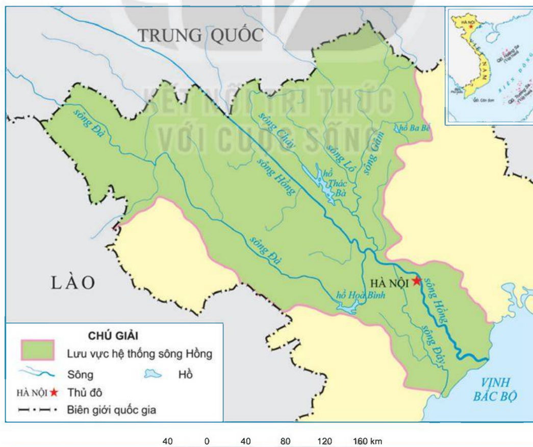
Hình 6.3. Lược đồ lưu vực hệ thống sông Hồng trên lãnh thổ Việt Nam
