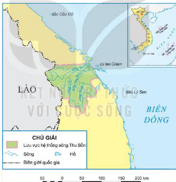
Hình 6.5. Lược đồ lưu vực hệ thống sông Thu Bồn
