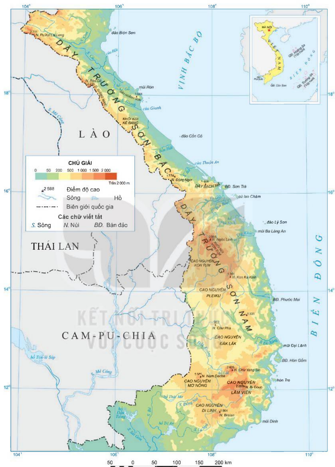
Hình 2.6. Lược đồ địa hình vùng núi Trường Sơn Bắc và vùng núi Trường Sơn Nam
