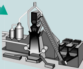
Lò luyện gang dùng không khí giàu oxy
