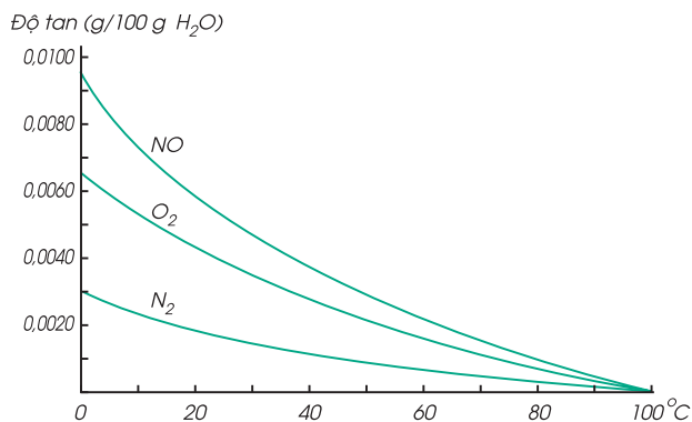
Hình 6.6 Ảnh hưởng của nhiệt độ đến độ tan của chất khí
