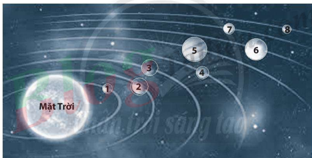
Hình 5.1. Trái Đất trong hệ Mặt Trời
