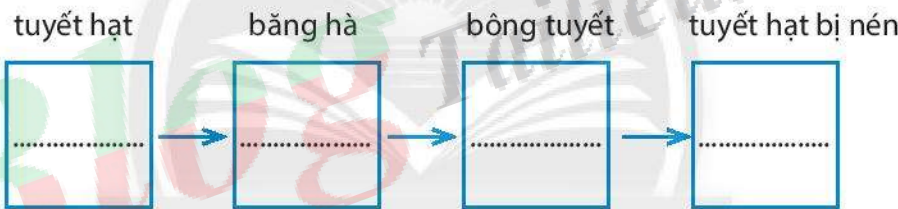
Hình 16.2. Quá trình hình thành băng hà
