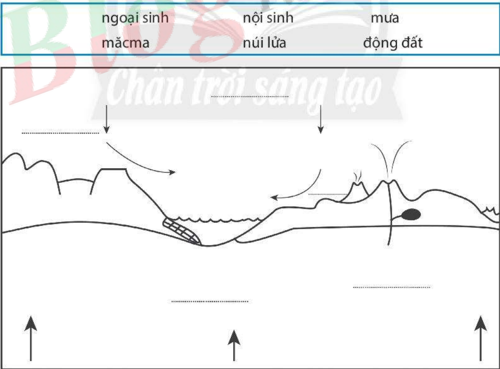
Hình 10.1. Quá trình nội sinh và ngoại sinh
