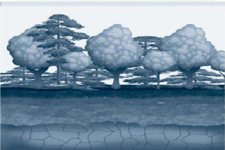
Hình 19.3. Đất ở vùng khí hậu nhiệt đới
