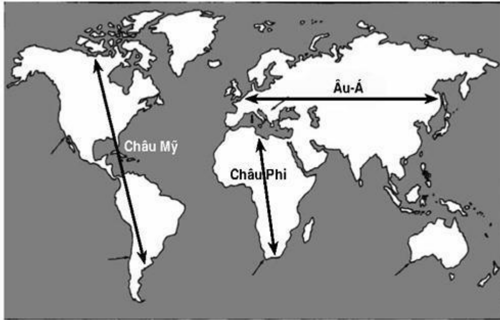
Hình 10.1: Trục chính của các lực địa
