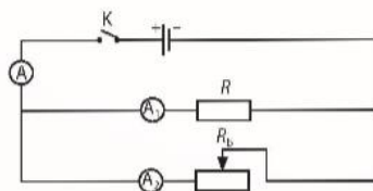
▲ Hình 10.3. Sơ đồ mạch điện mắc song song
