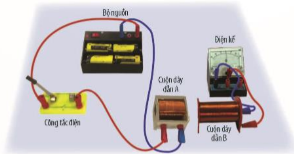
▲ Hình 12.2. Sơ đồ thí nghiệm dùng nam châm điện để tạo ra dòng điện
