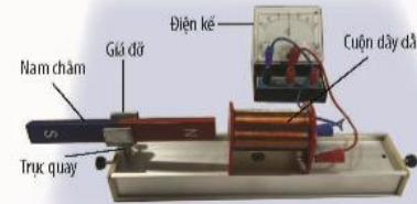
▲ Hình 12.1. Bô trí thí nghiệm dùng nam châm vĩnh cửu để tạo ra dòng điện
