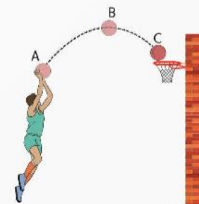
b) Quả bóng được ném vào rổ
