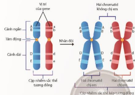
▲ Hình 41.3. Cặp nhiễm sắc thể tương đồng
