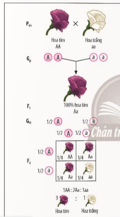
3.1. Thí nghiệm lai một cặp tính trạng màu sắc hoa ở đậu Hà lan của Mendel
