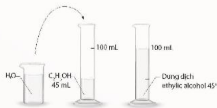
▲ Hình 24.2. Cách pha dung dịch ethylic alcohol 45^\circ
