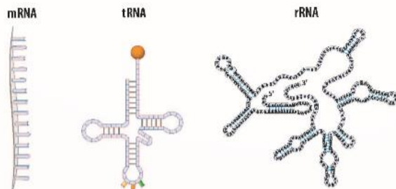
▲ Hình 37.2. Cấu trúc các phân tử RNA
