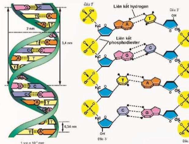
▲ Hình 37.1. Cấu trúc phân tử DNA
