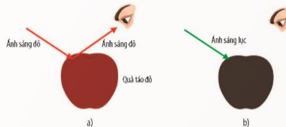
▲ Hình 5.7. a) Quả táo có màu đỏ dưới ánh sáng đỏ; b) Quả táo có màu gần như đen dưới ánh sáng lục
