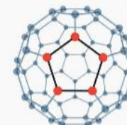
▲ Cấu trúc của fullerenes
