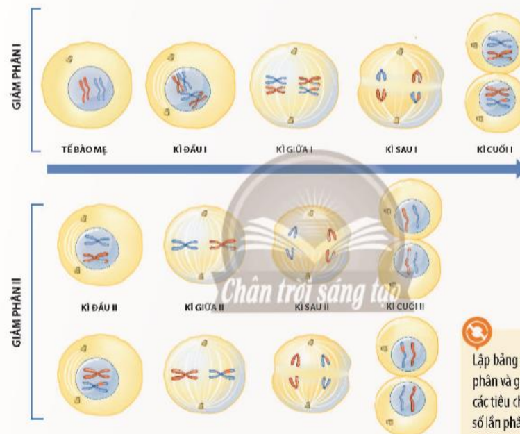
▲ Hình 43.2. Quá trình giảm phân
