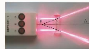
▲ Hình 7.9. Thí nghiệm với thấu kính phân kì:
