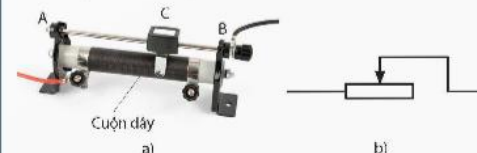
▲ a) Biến trở con chạy; b) Kí hiệu của biến trở trong mạch điện
