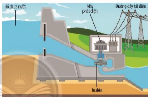
▲ Sơ đồ một đập thủy điện
