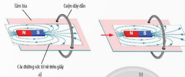
▲ Hình 12.5. Minh họa số đường sức từ xuyên qua tiết diện cuộn dây dẫn khi nam châm ở xa (a) và ở gần (b) cuộn dây dẫn
