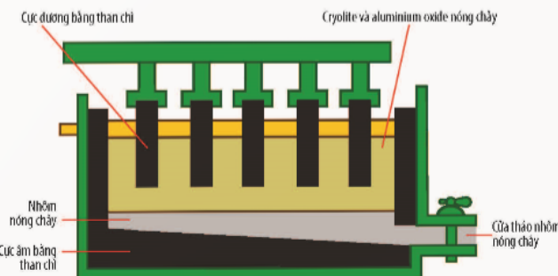
▲ Hình 17.4. Sơ đồ mô phỏng bể điện phân sản xuất nhôm
