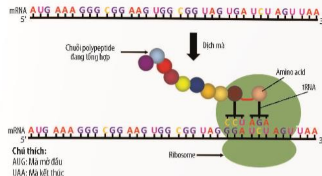
▲ Hình 39.4. Quá trình dịch mã
