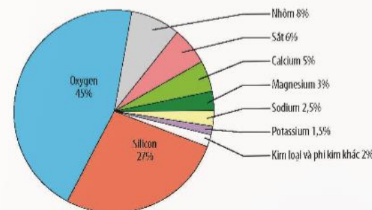
Hình 31.1. Thành phần phần trăm khối lượng các nguyên tố trong vỏ Trái Đất (*)
