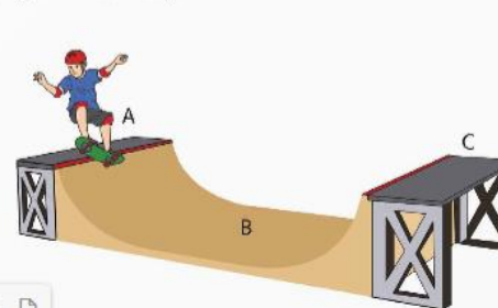
a) Một người trượt ván
