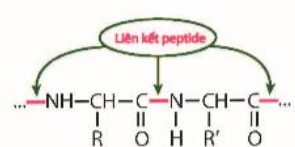
▲ Hình 29.2. Cấu tạo một đoạn mạch protein
