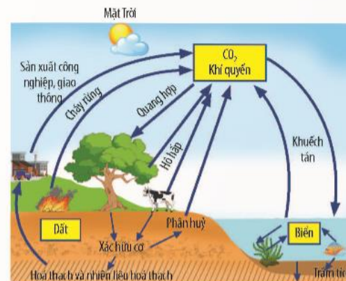
▲ Hình 14.2. Chu trình carbon trên Trái Đất
