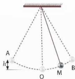
▲ Hình 2.4. Chuyển động của con lắc
