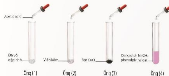
▲ Hình 25.4. Thí nghiệm acetic acid phản ứng với đá vôi, kẽm, copper(II) oxide, sodium hydroxide
