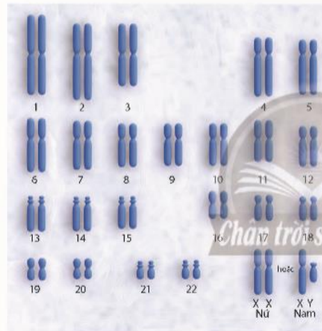
▲ Hình 43.5. Bộ nhiễm sắc thể ở người
