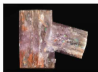
b) Khoáng vật calcite chứa \text{CaCO}_3
