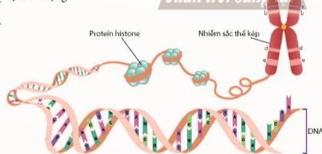
▲ Hình 41.5. Cấu trúc của nhiễm sắc thể
