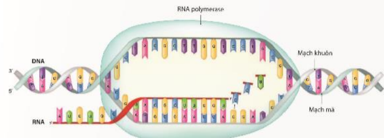
▲ Hình 39.3. Sơ đồ cơ chế phiên mã
