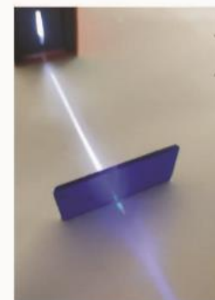
▲ Hình 5.8. Tấm lọc màu lam cho ánh sáng màu lam đi qua và hấp thụ hầu hết các ánh sáng màu còn lại
