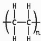
▲ Hình 30.1. Công thức cấu tạo polyethylene
