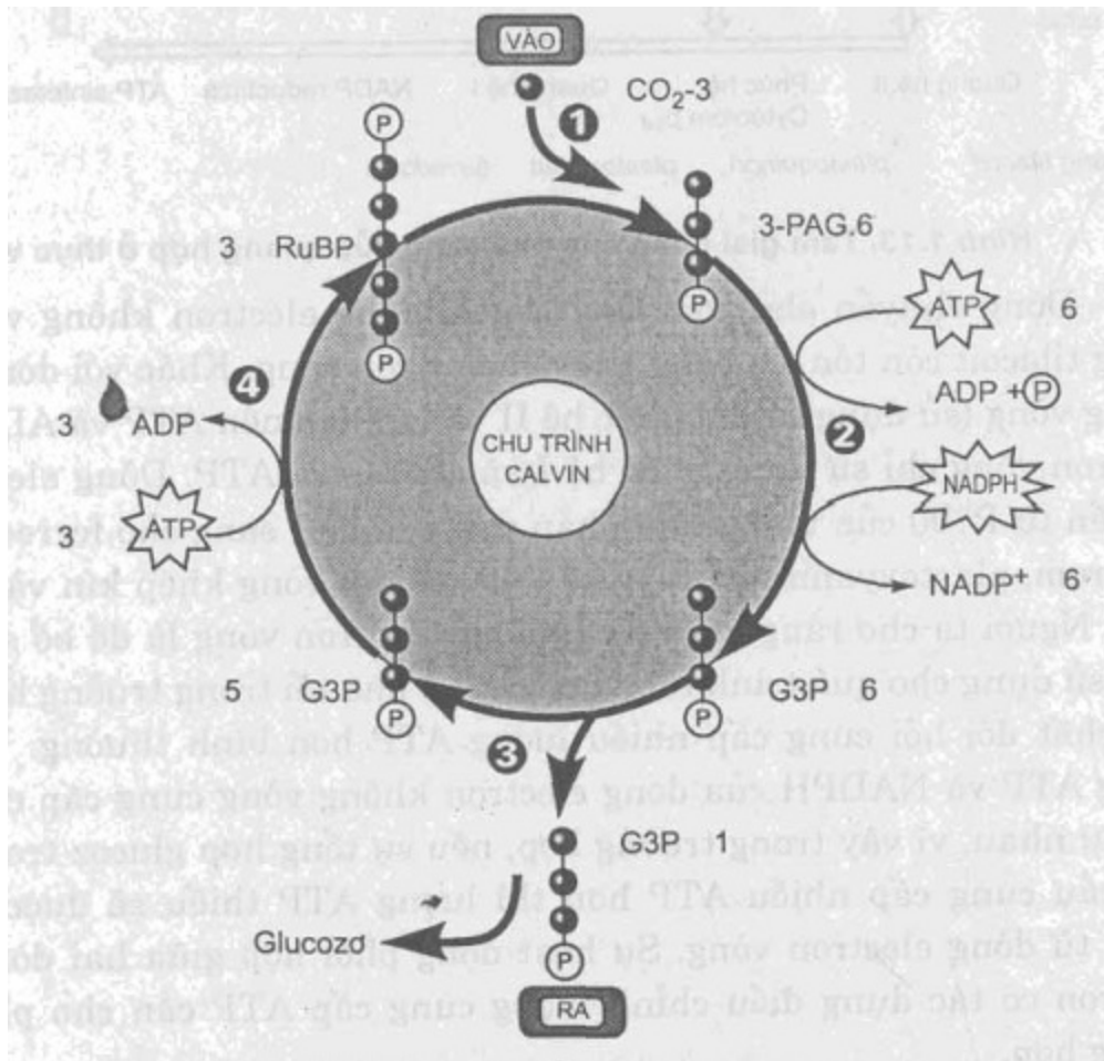
Hình 1.14. Sơ đồ tóm tắt chu trình Calvin
