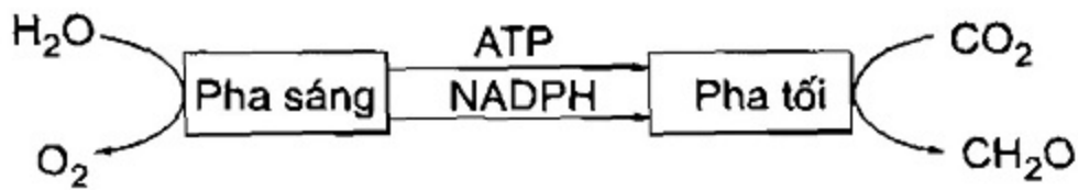
Hình 1.11. Sơ đồ 2 pha của quang hợp
