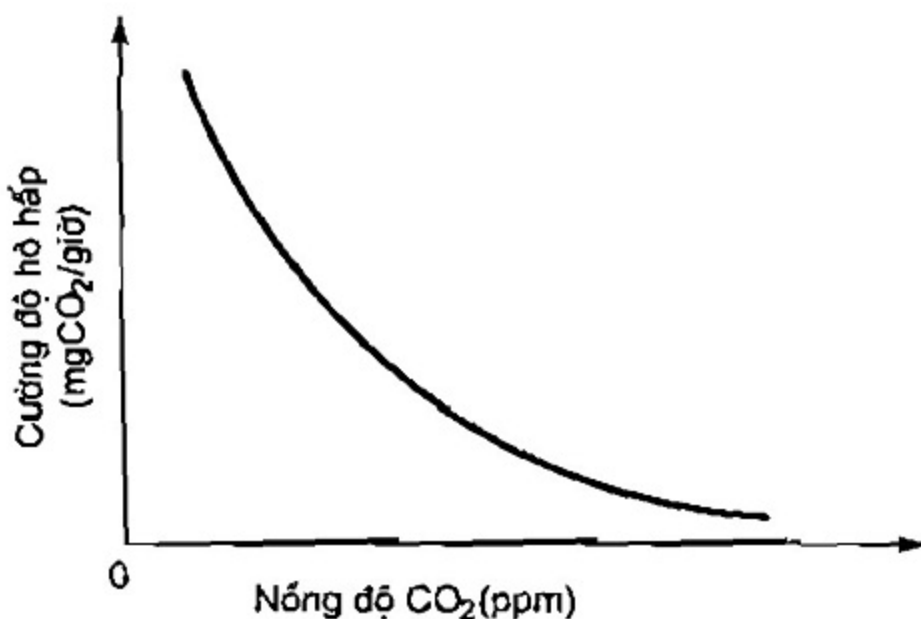
Hình 1.10. Ảnh hưởng của nồng độ \text{CO}_2 lên hô hấp.
