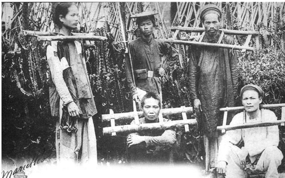
Nghĩa quân sa vào tay giặc Pháp Ba Đình
