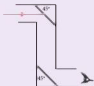
Hình 13.8. Sơ đồ kính tiềm vọng đơn giản
