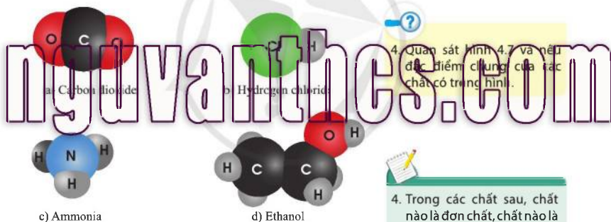
Hình 4.7. Mô hình phân tử của một số hợp chất
