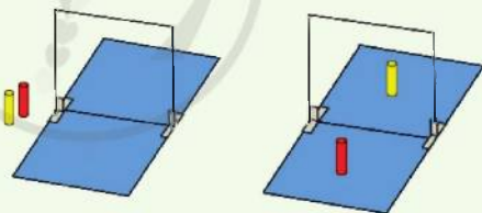
Hình 13.9. Hình vẽ gợi ý các bước tiến hành thí nghiệm kiểm chứng tính chất ảnh của vật qua gương phẳng
