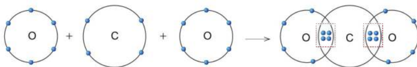
Hình 5.11*. Sơ đồ tạo thành liên kết trong phân tử carbon dioxide
