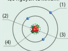
Hình 1.3. Mô hình cấu tạo nguyên tử lithium
