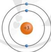
a) Lithium
