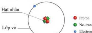
Hình 1.2. Mô hình cấu tạo nguyên tử helium
