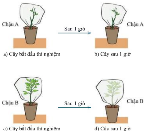
Hình 25.7. Sơ đồ minh họa thí nghiệm 1
