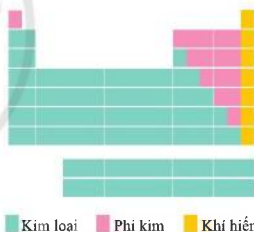
Hình 3.7. Vị trí của các nguyên tố kim loại, phi kim, khí hiếm trong bảng tuần hoàn
