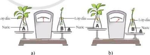
Hình 25.8. Sơ đồ minh họa thí nghiệm 2
