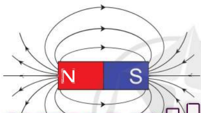
Hình 15.4. Đường sức từ của một thanh nam châm được vẽ theo quy ước
