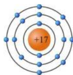
b) Chlorine
