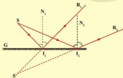
Hình 13.12. Ảnh S' của S qua gương phẳng
