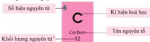
Hình 3.1. Ô nguyên tố carbon
