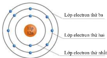
Hình 1.4. Mô hình cấu tạo nguyên tử sodium
