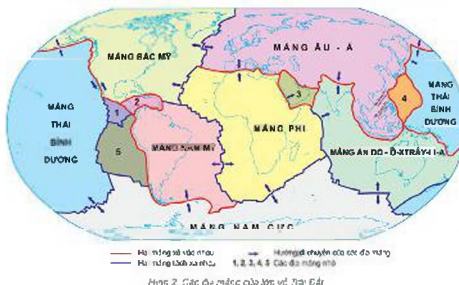
Hình 2. Các địa mảng của lớp vỏ Trái Đất
