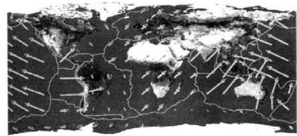
Plate movement Sự di chuyển của phiến lục địa
