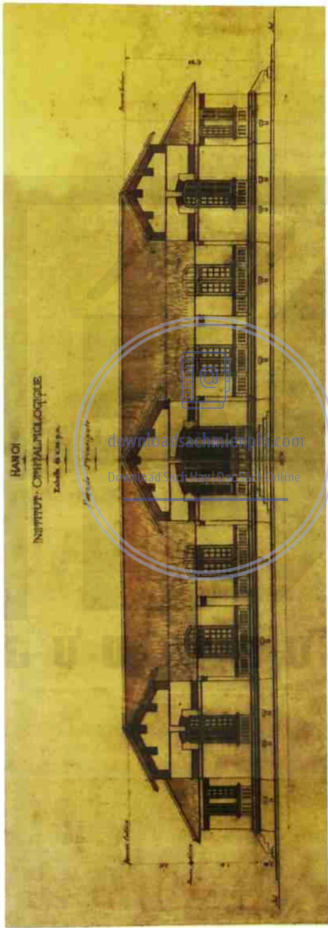
Bản vẽ mặt trước Viện Mắt (nay là Viện Mắt Trung ương) do kiến trúc sư Adolphe Bussy, Chánh Sở Nhà cửa dân sự lập 1914, tỷ lệ 1/50, kích thước gốc 28cm x 80cm. KT - 539/1.
