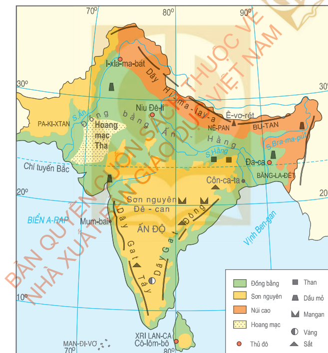
Hình 10.1. Lược đồ tự nhiên khu vực Nam Á
