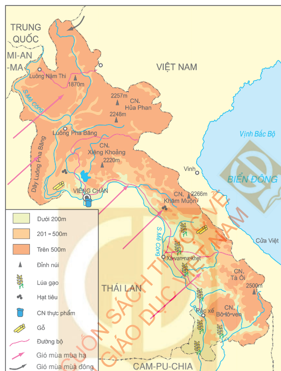
Hình 18.2. Lược đồ tự nhiên, kinh tế Lào
