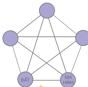
Hình 20.5. Sơ đồ mối quan hệ giữa các thành phần tự nhiên
