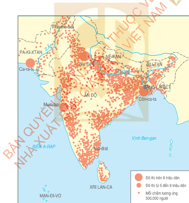
Hình 11.1. Luộc đồ phân bố dân cư Nam Á
