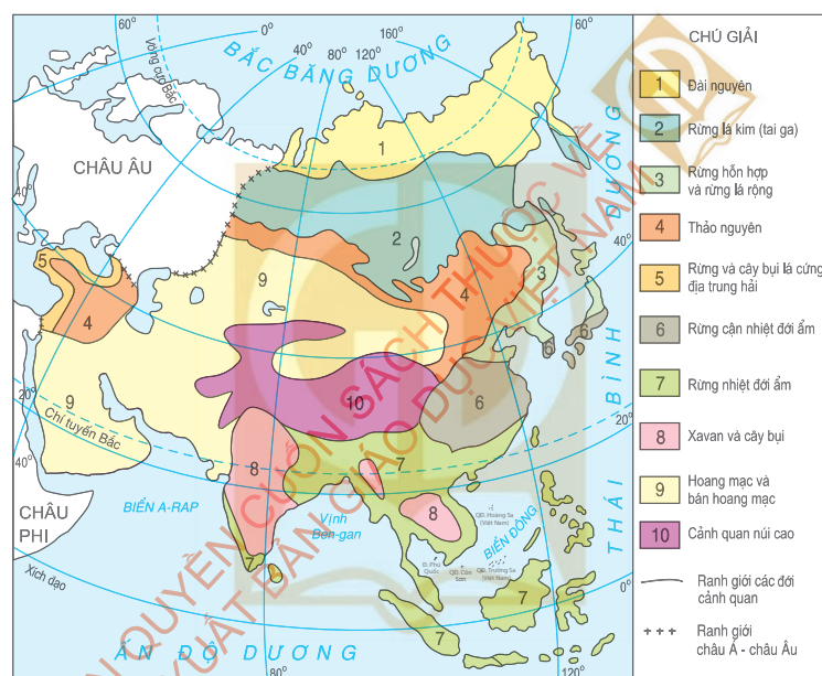
Hình 3.1. Luộc đồ các đới cảnh quan tự nhiên châu Á
