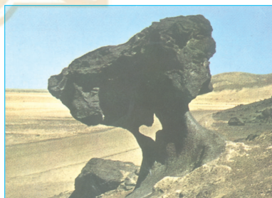
b) Nấm đá ba dan ở Ca-li-phoóc-ni-a (Hoa Kỳ)
