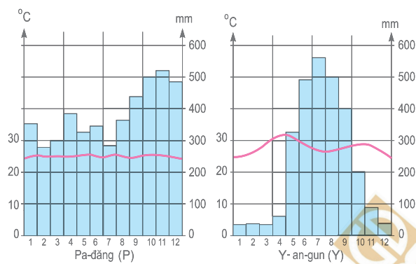
Hình 14.2. Biểu đồ nhiệt độ và lượng mưa
