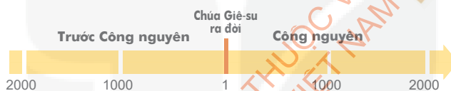
▲ Hình 3. Sơ đồ cách tính thời gian theo Công lịch
