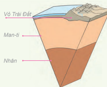
Hình 1. Lát cắt về cấu tạo Trái Đất
