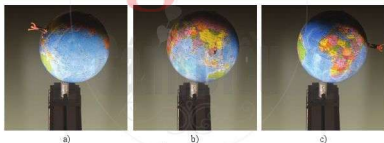
Hình 33.3. Mô hình Trái Đất quay quanh trục từ phía tây sang phía đông
