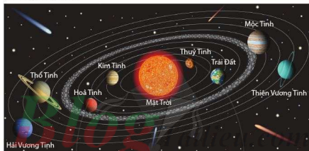
Hình 35.3. Hệ Mặt Trời
