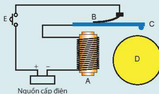
Hình 20.4 Sơ đồ cấu tạo chuông điện
