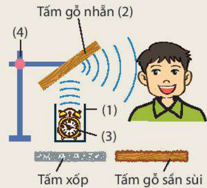
Hình 14.3 Bố trí thí nghiệm phản xạ âm
