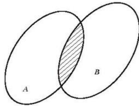
A \cap B Hình 5
