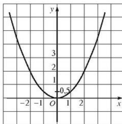
Đồ thị hàm số g(x) = \frac{1}{2}x^2
