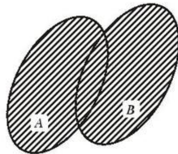
A \cup B Hình 6
