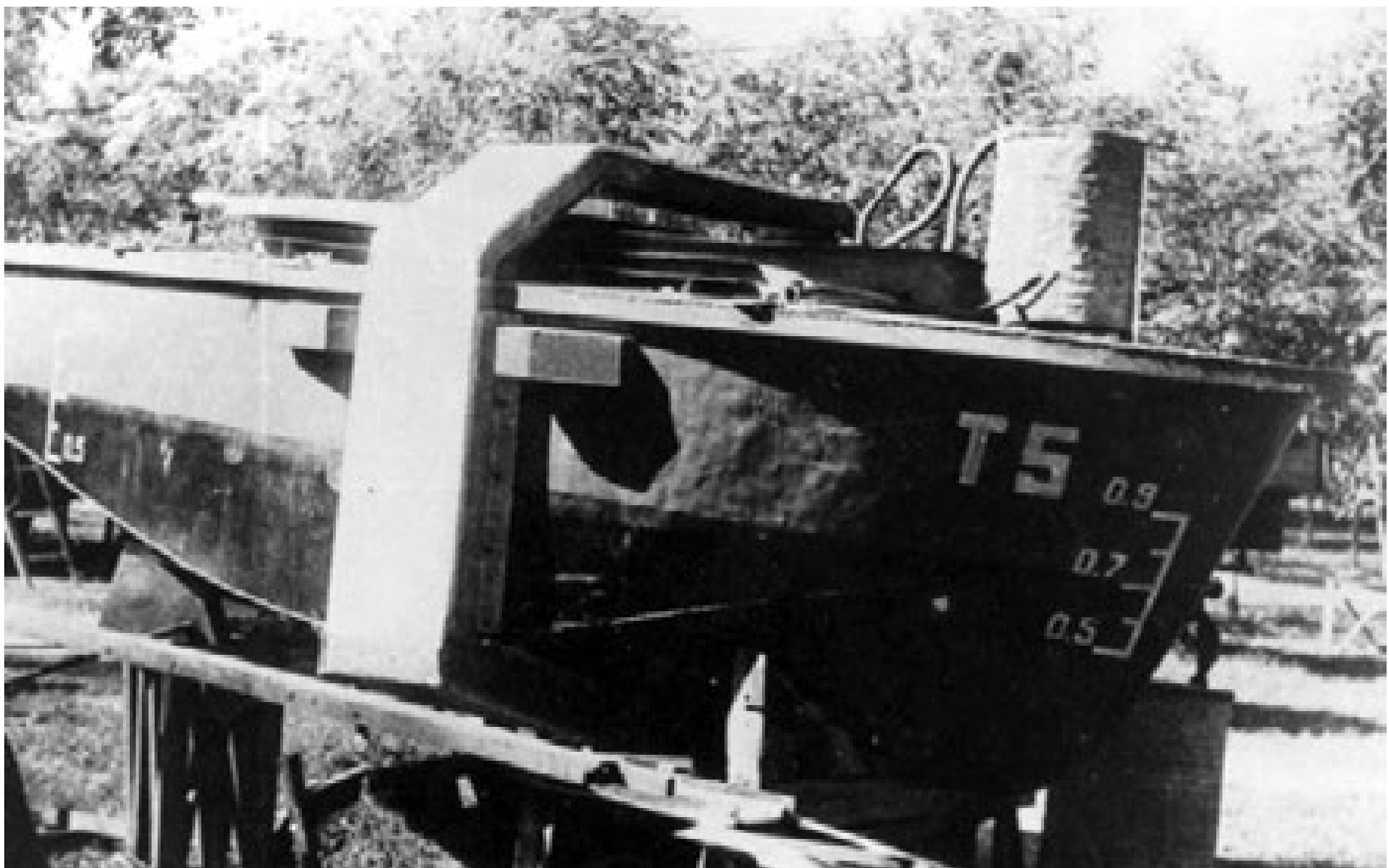
Tàu T5, loại tàu phá thủy lôi điều khiển từ xa.
