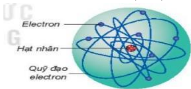
Hình 3.1. Mô hình hành tinh nguyên tử của E. Rutherford (Rô-đô-phô), N. Bohr (Bo) và A. Sommerfeld (Zôm-mô-phen)
