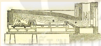
Hình 10. Lò luyện quặng theo phương pháp “put-đinh” (Hen-ri Côt)
