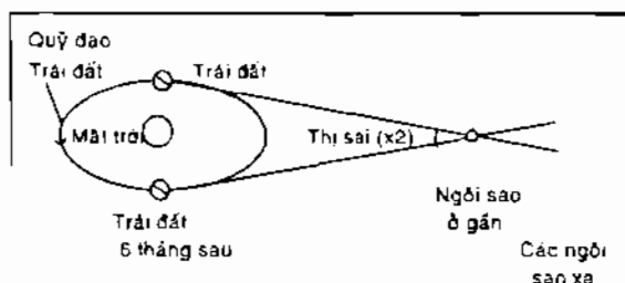
Hình 5. Phép đo khoảng cách tới các ngôi sao.
