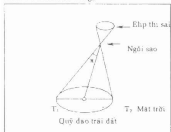
Hình 3. Thị sai hằng năm của một ngôi sao
