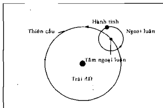
Hình 1. Vũ trụ của Ptolômê. Để giải thích chuyển động của mỗi hành tinh, Ptolômê đã cho mỗi hành tinh chuyển động trên một vòng tròn nhỏ gọi là ngoại luân. Tâm của vòng tròn này quay trên thiên cầu có tâm ở Trái đất.
