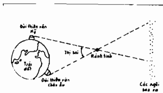
Hình 4. Đo khoảng cách tới các hành tinh
