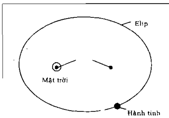
Hình 2. Elip Kepple
