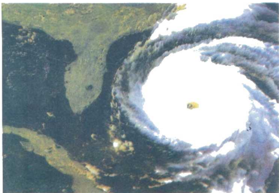
Một cơn bão nhìn từ vệ tinh
