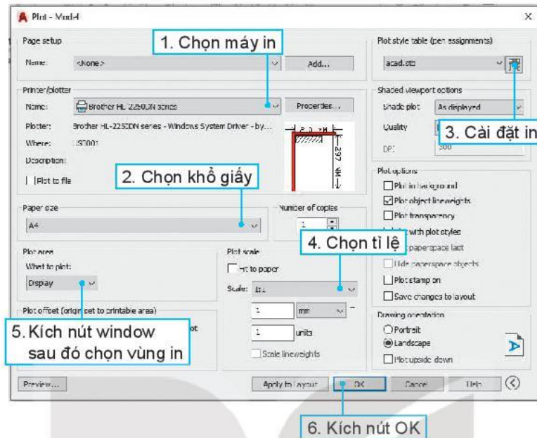
Hình 3.8. Điều khiển in
