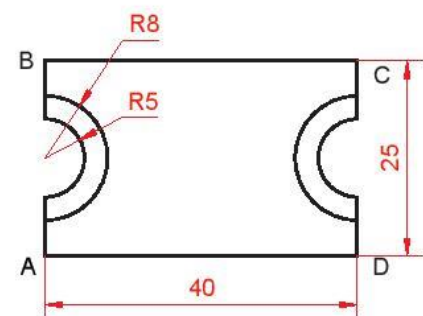
Hình 2.8. Tấm đế
