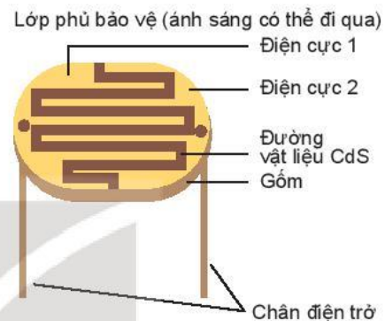
Hình 5.8. Cấu tạo của quang trở
