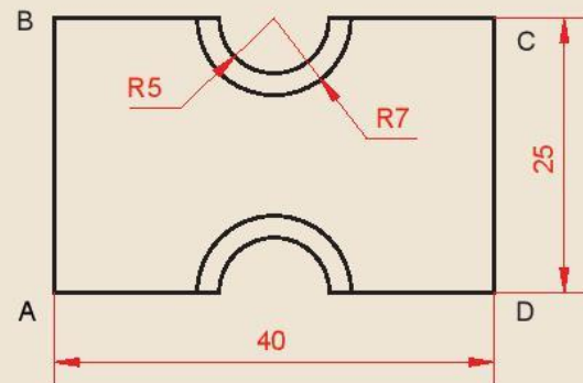
Hình 2.10. Tấm đế
