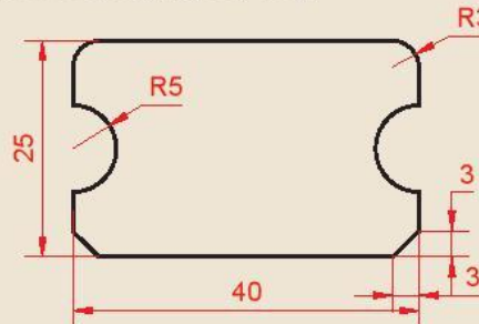
Hình 2.6. Tấm đỡ
