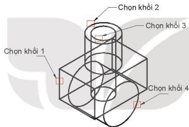
Hình 2.23. Chọn để liên kết các khối
