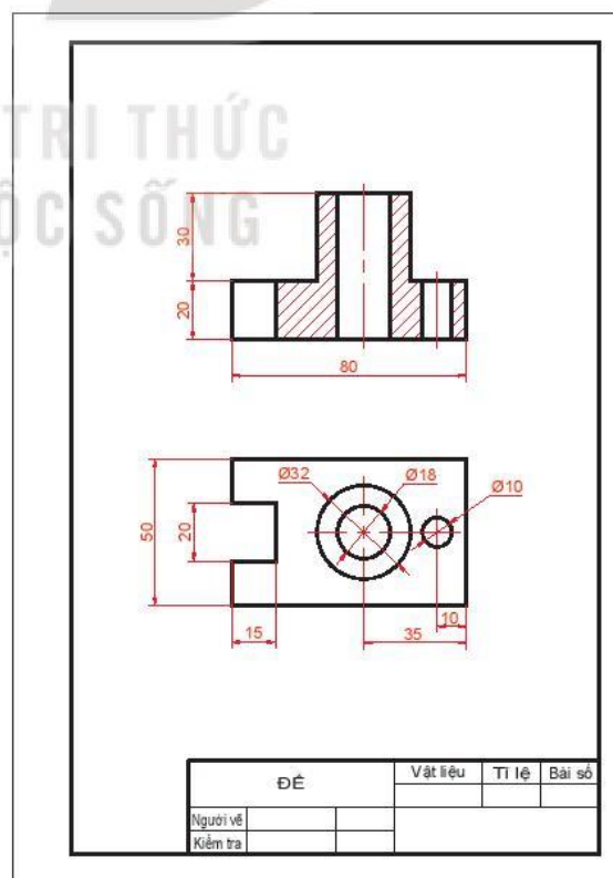
Hình 3.2. Bản vẽ cái đế
