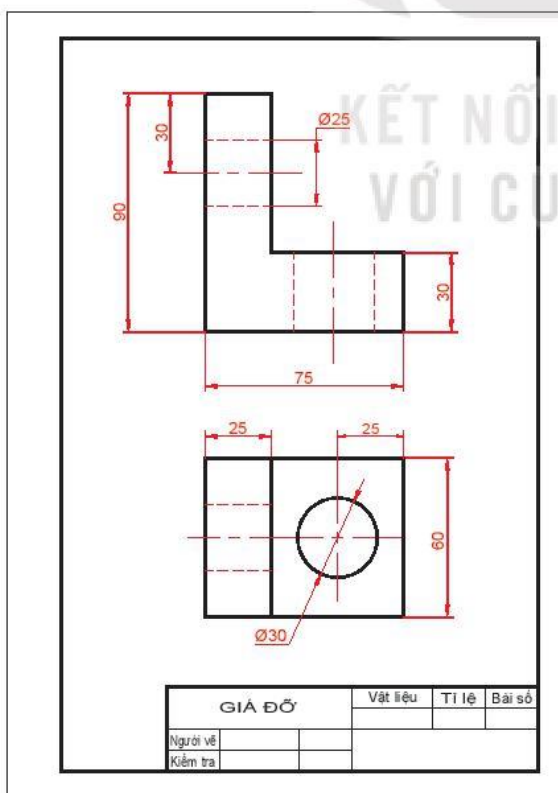
Hình 3.1. Bản vẽ giá đỡ
