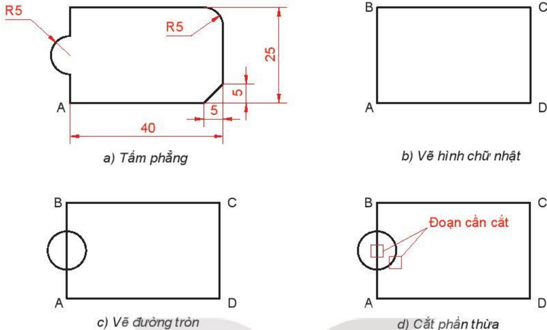
Hình 2.5. Sử dụng các lệnh hiệu chỉnh
