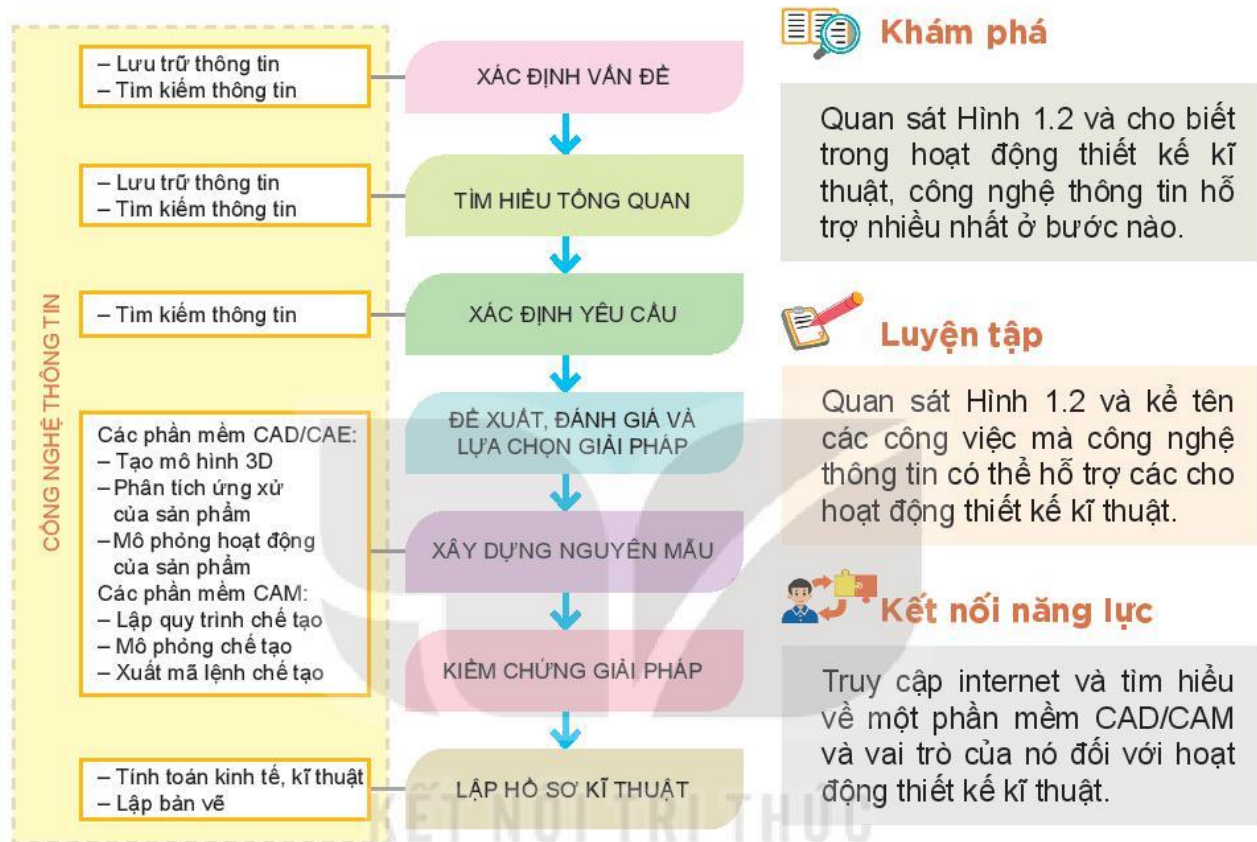
Hình 1.2. Vai trò công nghệ thông tin trong quy trình thiết kế kỹ thuật
