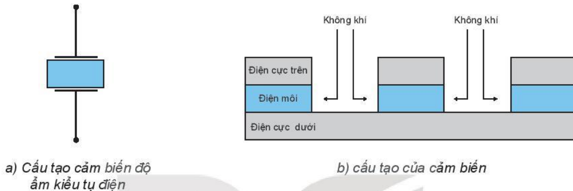
Hình 5.5. Cấu tạo của cảm biến độ ẩm kiểu tụ điện
