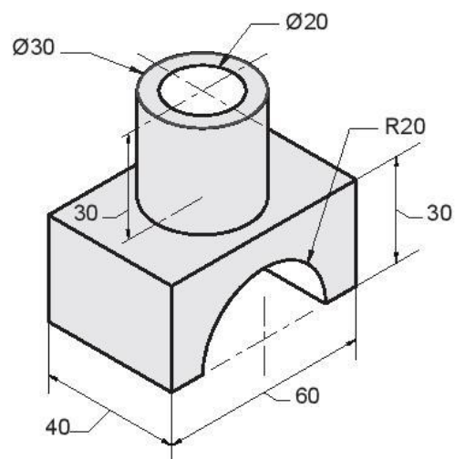
Hình 2.17. Giá đỡ
