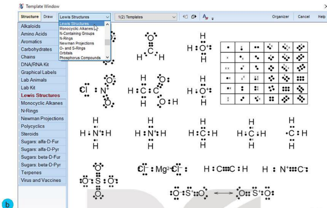
Hình 9.4. Các bước vẽ công thức Lewis:
