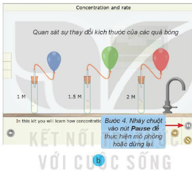
Hình 10.3. Các bước mô phỏng thí nghiệm về ảnh hưởng của nồng độ lên tốc độ phản ứng
