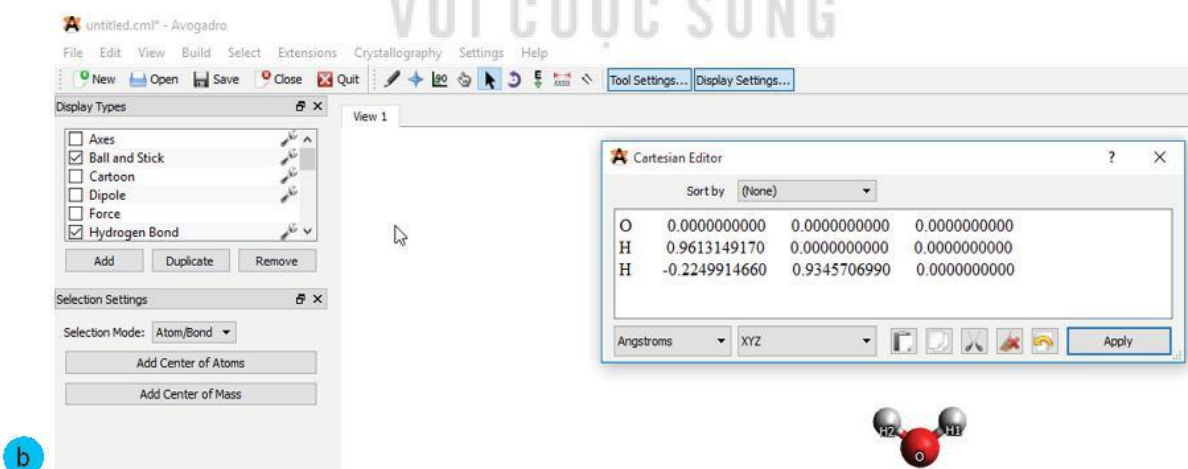
Hình 11.1. Cách hiển thị cấu trúc của phân tử H 2 O trong Avogadro từ kết quả tính tối ưu cấu trúc hình học sử dụng phần mềm MOPAC a) Cách hiển thị bằng tọa độ Descartes; b) Cách dán tọa độ vào bảng tọa độ Descartes để hiển thị cấu trúc.
