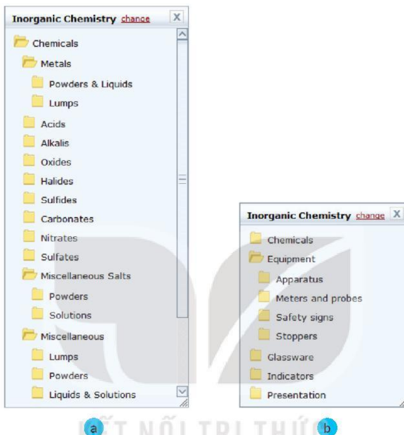
Hình 10.4. a) Giao diện hoá chất; b) giao diện thiết bị và dụng cụ thí nghiệm.
