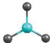
Mô hình phân tử AX_3
