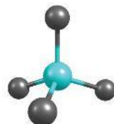
Mô hình phân tử AX_4
