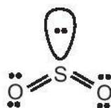
Sơ đồ phân tử SO_2
