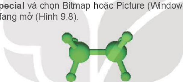
Hình 9.8. Ảnh cấu trúc phân tử C_2H_6 dạng Bitmap
