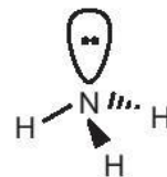
Sơ đồ phân tử NH_3
