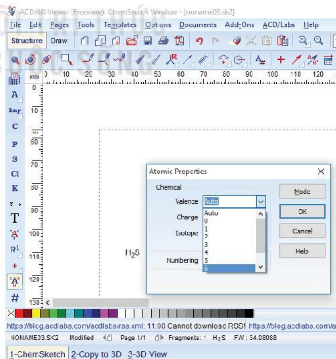
Hình 9.3. Thao tác chọn hoá trị
