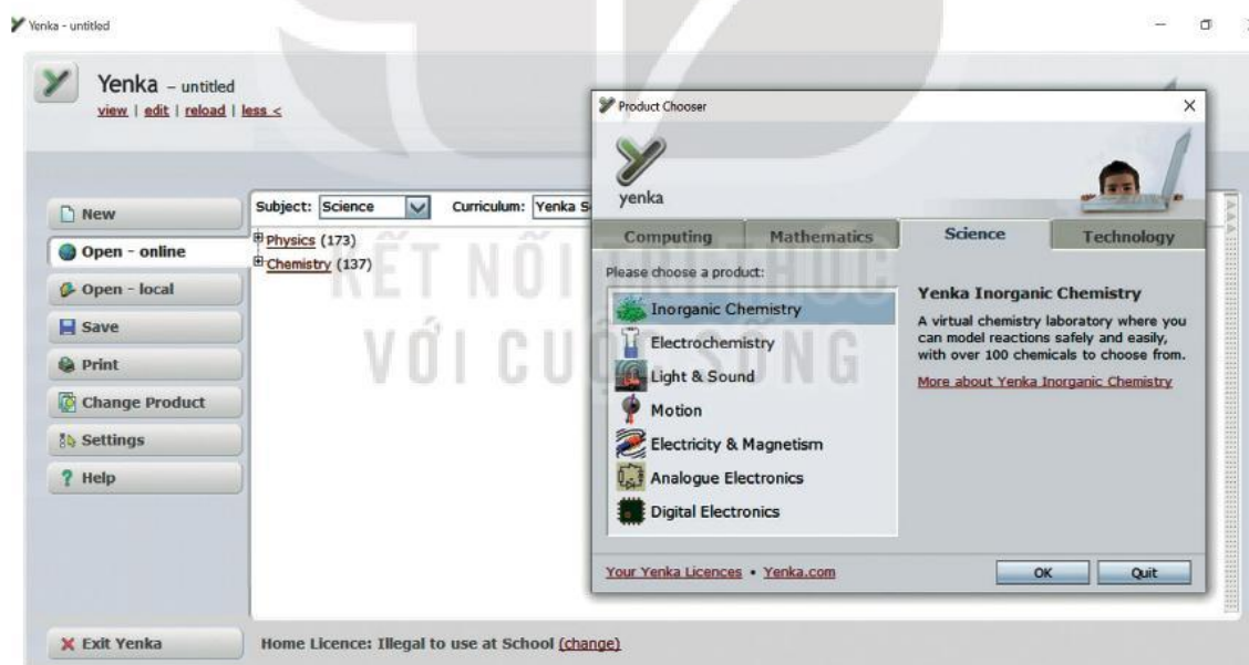
Hình 10.1. Giao diện của phần mềm Yenka
