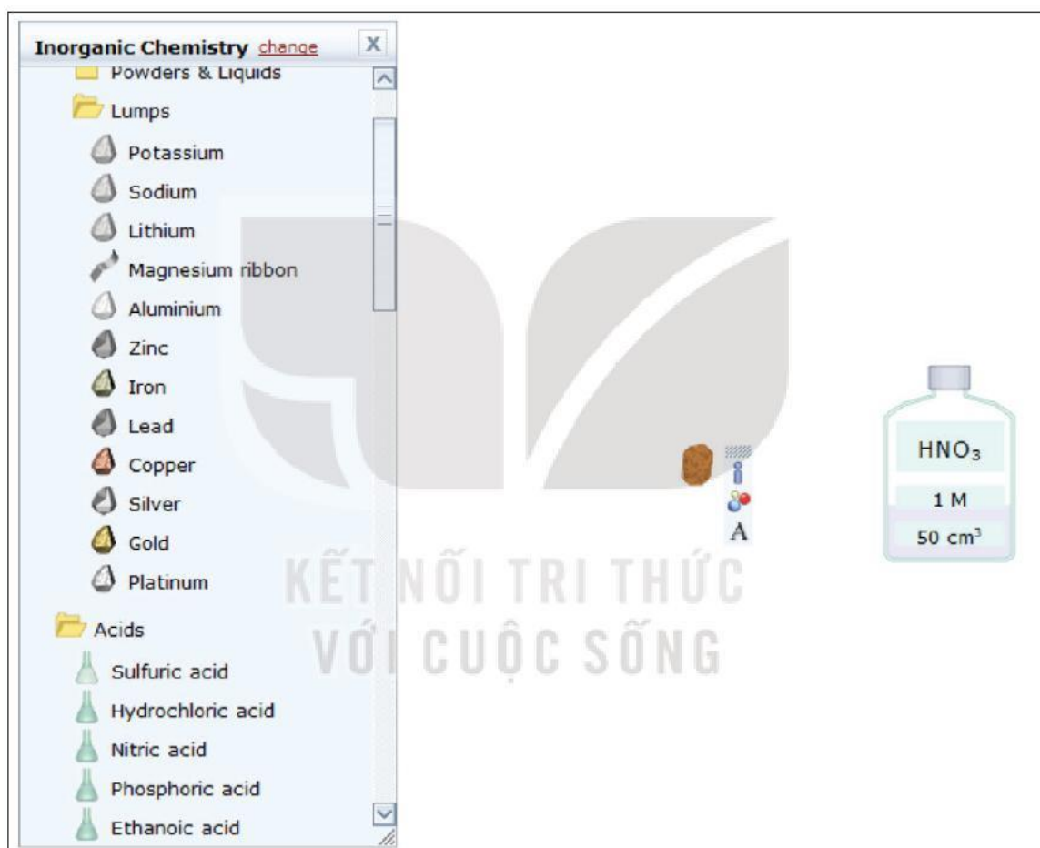
Hình 10.5. Chọn hoá chất copper và nitric acid
