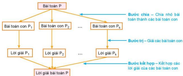
Hình 6.2. Sơ đồ ý tưởng chia để trị
