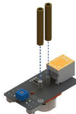
Hình 4.12. Lắp trụ đồng vào bánh đa hướng và cảm biến siêu âm
