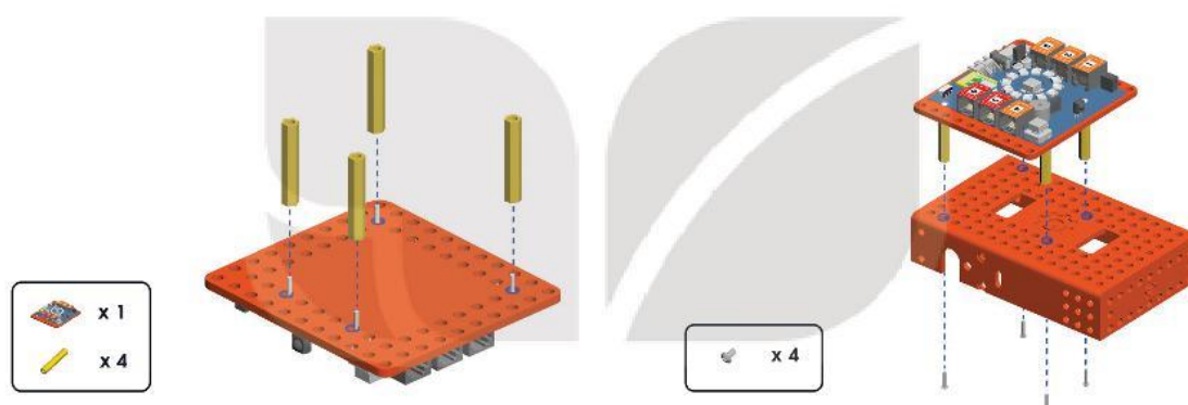
Hình 4.1. Lắp trụ đồng
