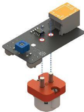
Hình 4.11. Lắp ghép cảm biến dò đường vào bánh đa hướng
