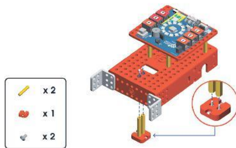
Hình 4.5. Lắp 2 trụ đồng và bánh đĩa hướng vào dưới thân 9×15
