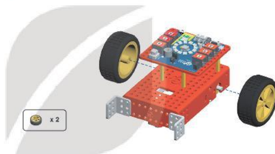
Hình 4.7. Lắp 2 bánh xe
