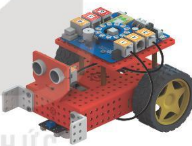
Hình 4.16. Sản phẩm sau khi hoàn thành
