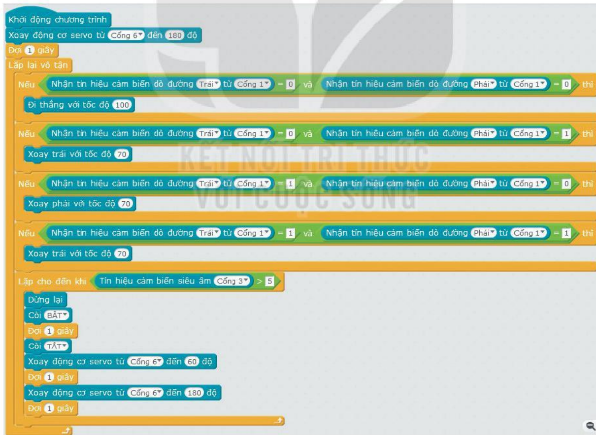
Hình 14.10. Chương trình hoàn chỉnh để robot thiện thực hiện nhiệm vụ 2
