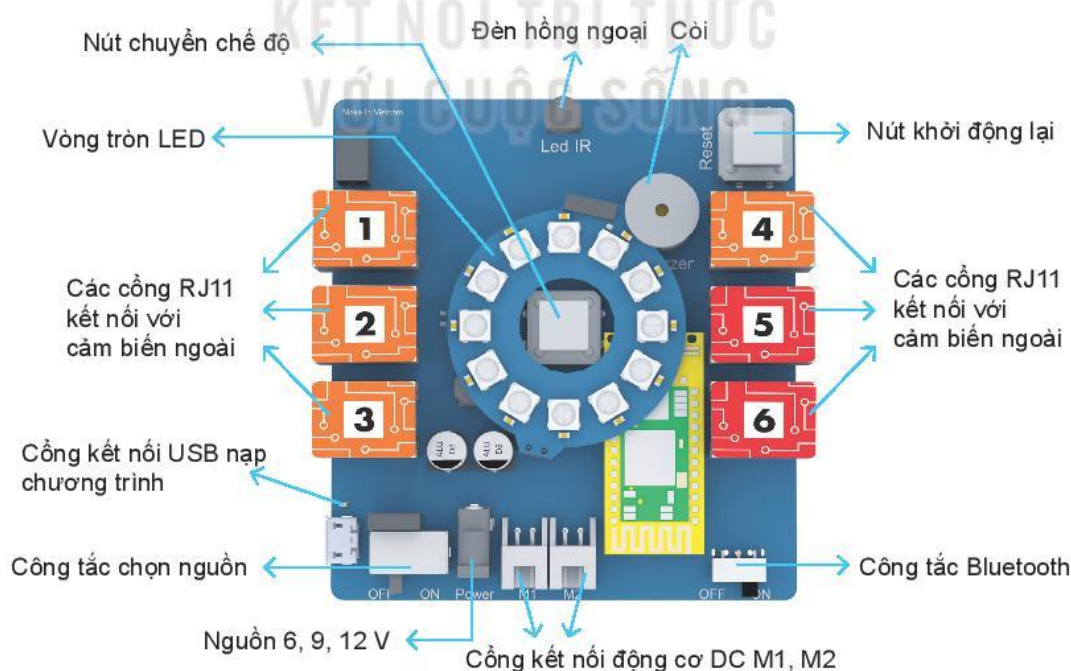
Hình 2.2. Bảng mạch điều khiển của G-Robot
