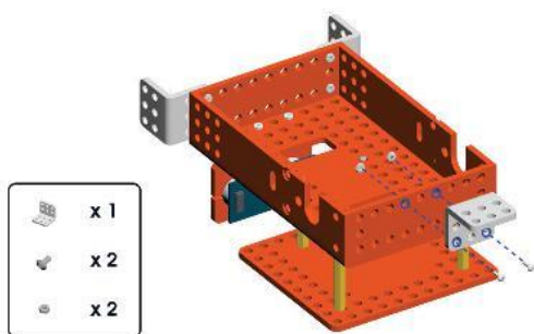
Hình 4.4. Lắp tấm vuông L 2×2×3 vào sau thân 9×15
