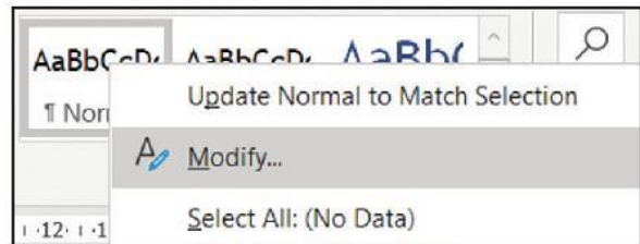
Hình 1.6. Lệnh Modify
