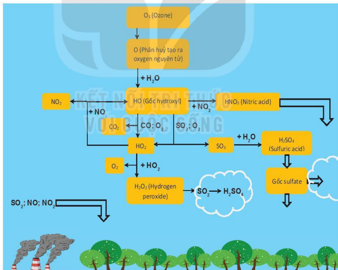
Hình 9.4. Quá trình mưa acid
