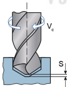
Hình 8.5. Thông số chế độ cắt khi khoan
