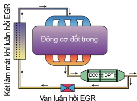
Hình 20.11. Hệ thống luân hồi EGR kết hợp bộ DOC và DPF
