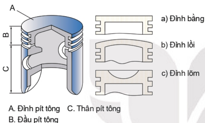
Hình 19.3. Cấu tạo
