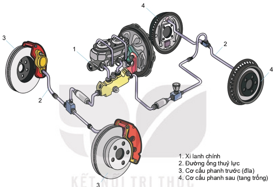
Hình 25.2. Hệ thống phanh trên ô tô con
