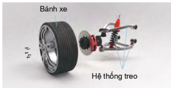
Hình 21.5. Bánh xe và hệ thống treo
