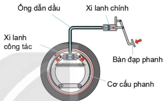
Hình 21.6. Hệ thống phanh
