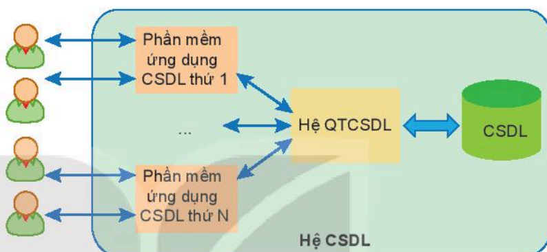
Hình 12.3. Hệ cơ sở dữ liệu
