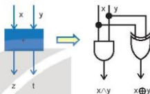
Hình 4.10. Mạch logic thực hiện phép cộng
