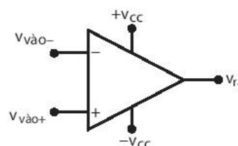
Hình 8.2 a. Kí hiệu bộ khuếch đại thuật toán. V_{\text{vào}+} lối vào không đảo, V_{\text{vào}-} lối vào đảo, +V_{\text{cc}} chân nguồn dương, -V_{\text{cc}} chân nguồn âm, V_{\text{ra}} chân ra
