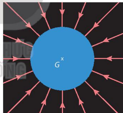
Hình 2.2. Biểu diễn đường sức trường hấp dẫn
