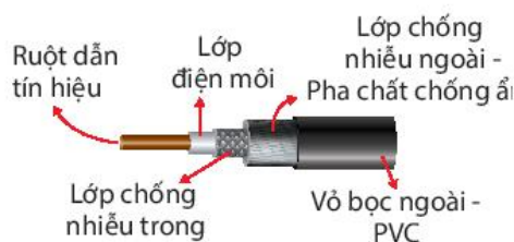
b) Cáp đồng trục
