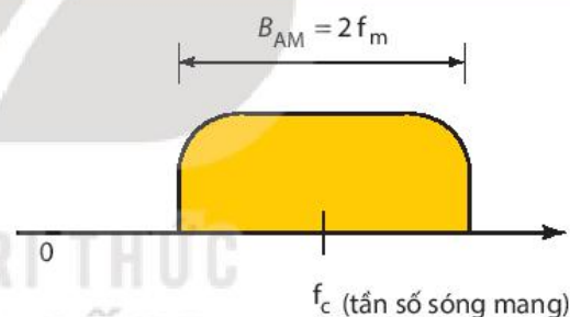
Hình 4.3. Băng thông của tín hiệu biến điệu
