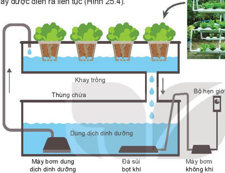
Hình 25.4. Hệ thống thủy canh hồi lưu
