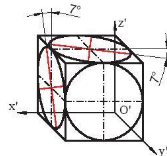
Hình 11.11. Các elip trong HCTĐ xiên góc cân
