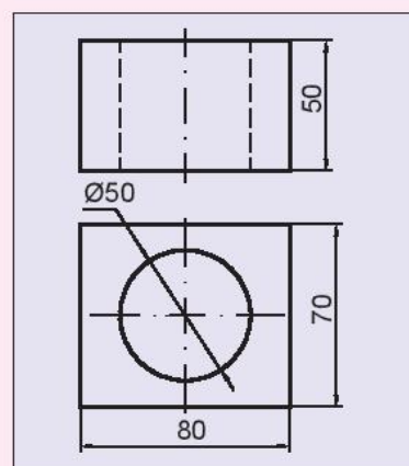
Hình 8.11. Giá đỡ
