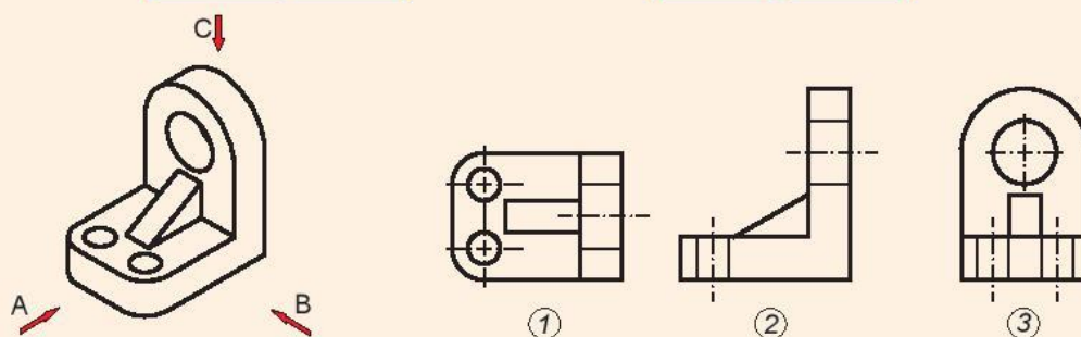
Hình 9.9. Gối đỡ
