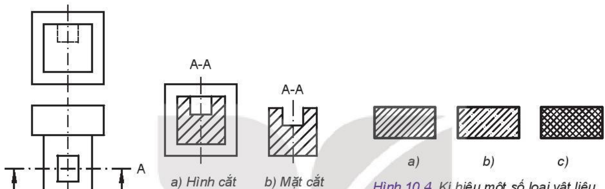
Hình 10.4. Kí hiệu một số loại vật liệu
