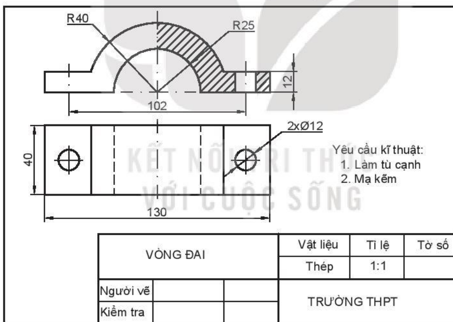
Hình 14.7. Bản vẽ chi tiết vòng đai
