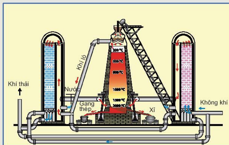
Hình 3.2. Sản xuất gang – thép trong lò cao
