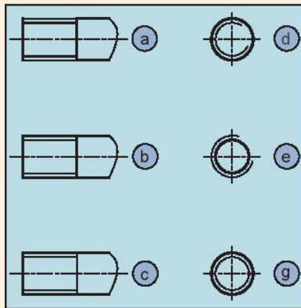
Hình 13.8. Ren trục
