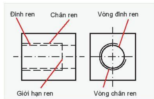
Hình 13.7. Ren khuất
