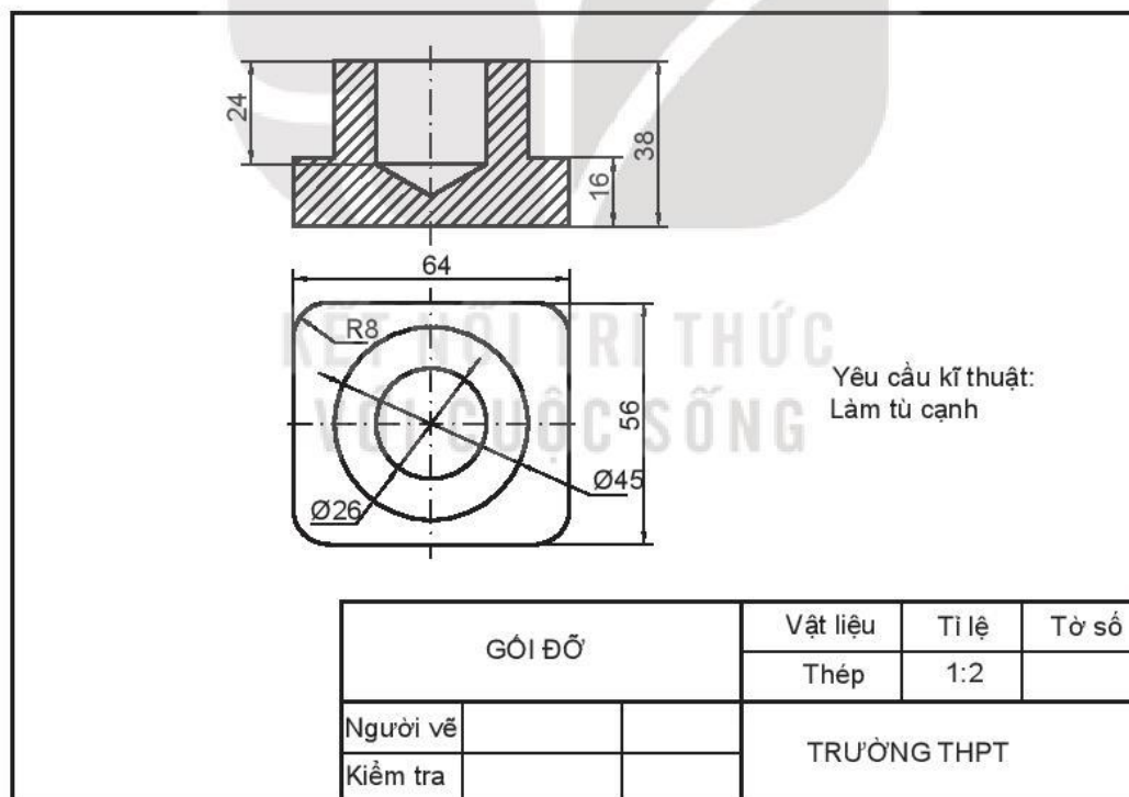
Hình 14.2. Bản vẽ gói đỡ
