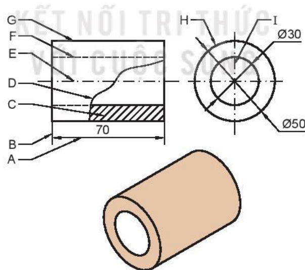
Hình 8.7. Bạc đỡ
