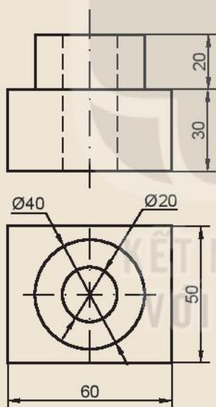
Hình 11.18. Gối đỡ
