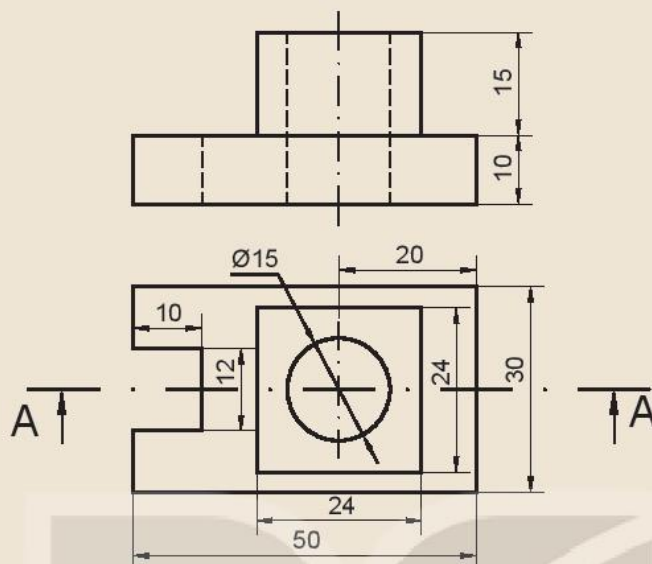
Hình 10.16. Đế
