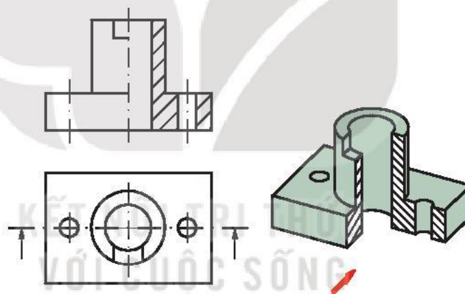
Hình 10.7. Hình cắt một nửa
