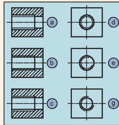
Hình 13.9. Ren lỗ
