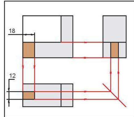
Hình 9.14. Vẽ rãnh hình hộp
