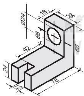
Hình 9.10. Giá đỡ
