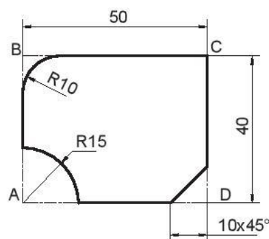
Hình 16.5. Tấm phẳng
