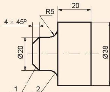
Hình 16.4. Trục
