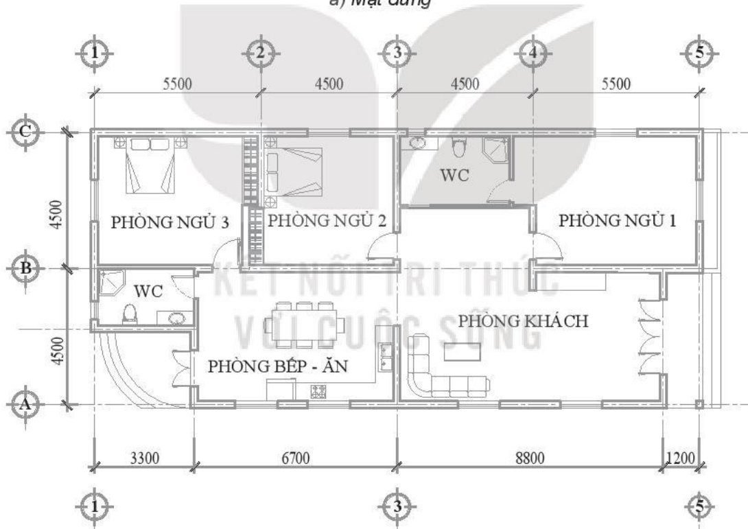
b) Mặt bằng
