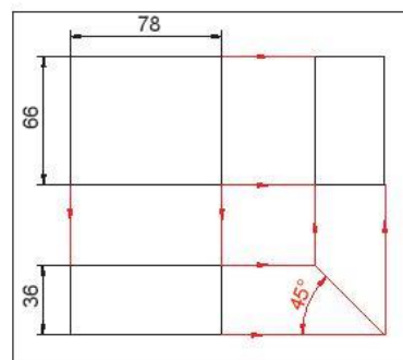
Hình 9.11. Phân tích vật thể thành các hình đơn giản và chọn các hướng chiếu
