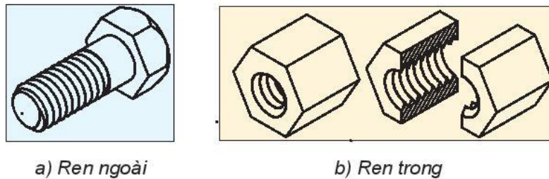
Hình 13.3. Ren ngoài và ren trong
