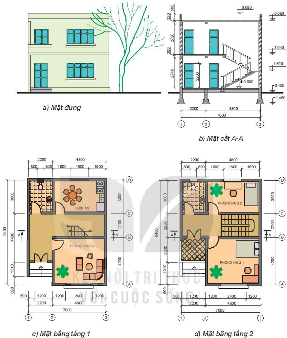
Hình 15.3. Bản vẽ nhà hai tầng
