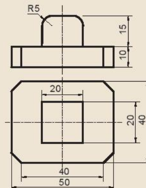
Hình 16.7. Gối đỡ
