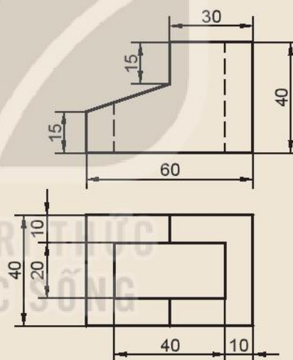
Hình 11.19. Đế
