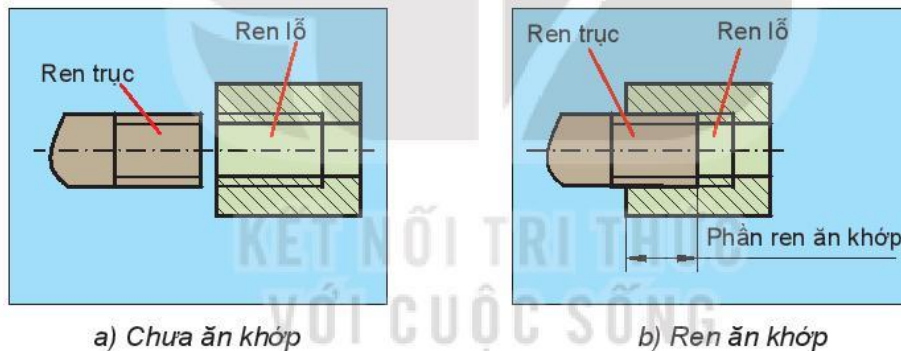
Hình 13.11. Ren ăn khớp
