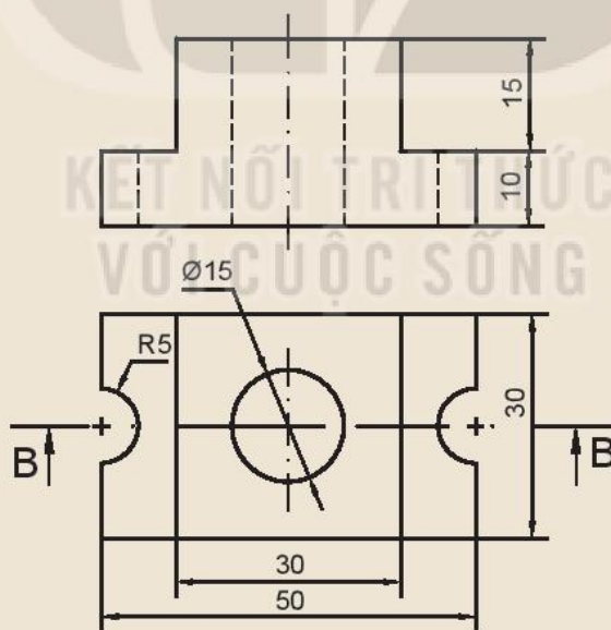
Hình 10.17. Gối đỡ
