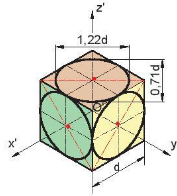
Hình 11.6. Các elip trong HCTĐ vuông góc đều
