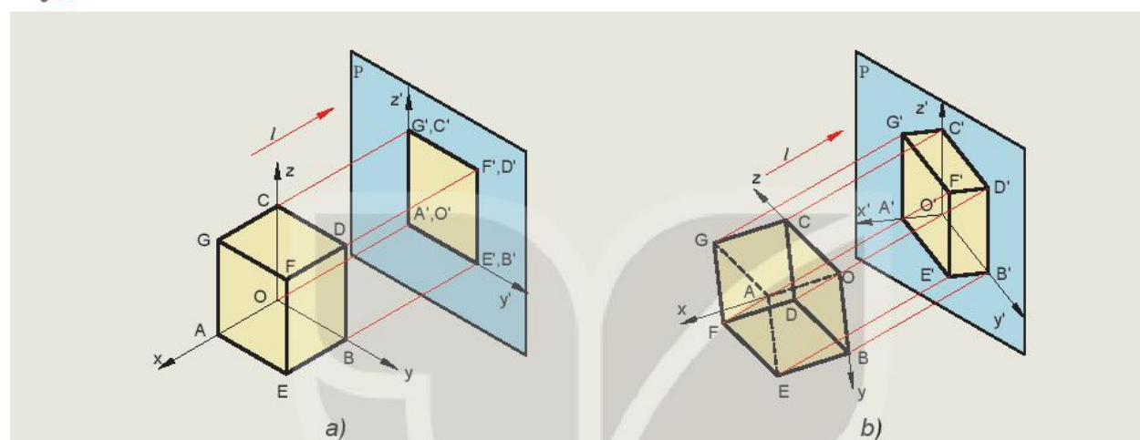
Hình 11.3. Vị trí hệ toạ độ ảnh hưởng đến hình chiếu của vật thể
