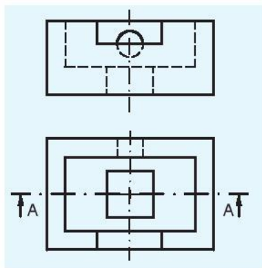
Hình 10.10. Giá đỡ
