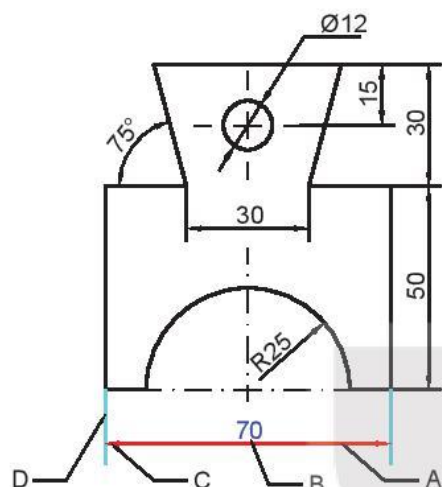
Hình 8.9. Giá đỡ
