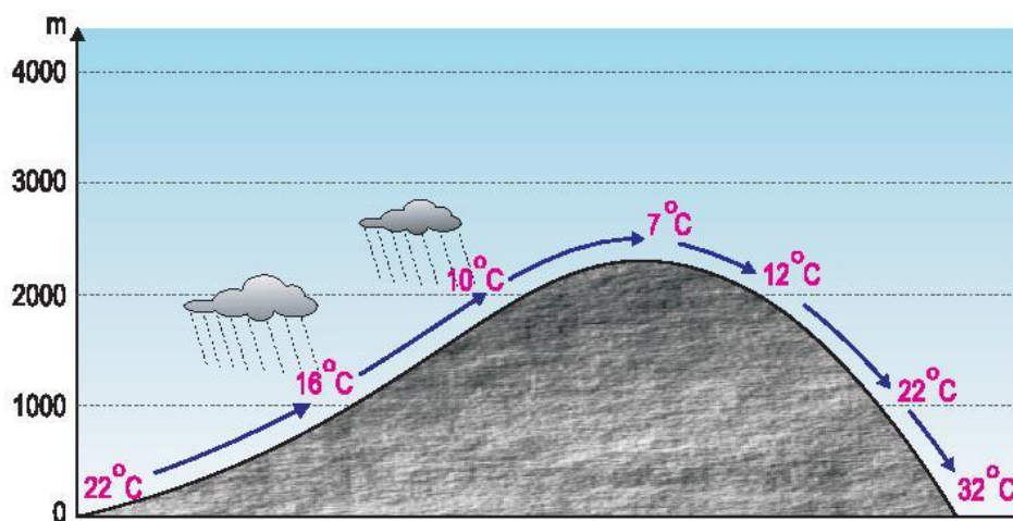
Hình 9.6. Gió fơn
