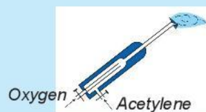
Hình 15.1. Sơ đồ cấu tạo đèn xì oxygen – acetylene
