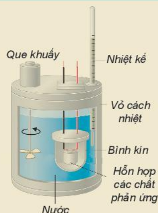
Hình 17.2. Một mô hình nhiệt lượng kế
