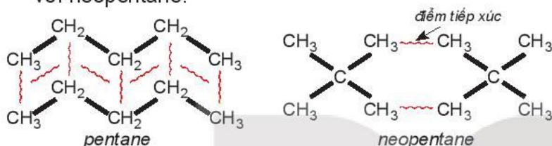
Hình 13.5. Tương tác van der Waals giữa các phân tử pentane và neopentane
