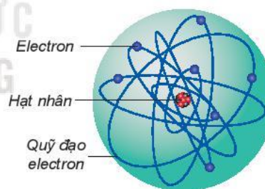
Hình 3.1. Mô hình hành tinh nguyên tử của E. Rutherford (Ro-do-pho), N. Bohr (Bo) và A. Sommerfeld (Zom-mo-phen)
