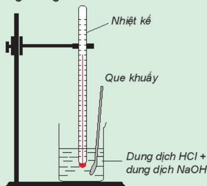
Hình 17.1. Theo dõi sự thay đổi nhiệt độ của phản ứng trung hoà
