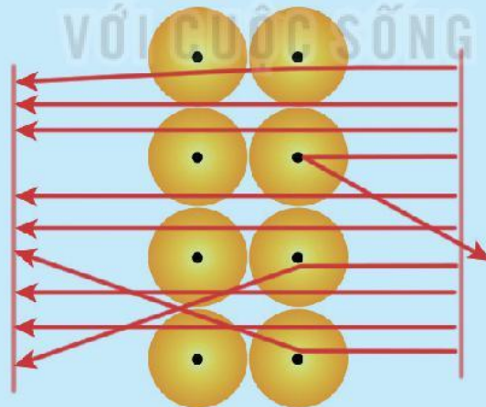
Hình 1.3. Mô phỏng kết quả thí nghiệm bắn phá lá vàng
