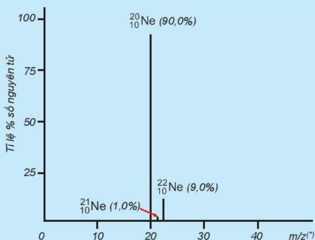
Hình 2.4. Phổ khối lượng của neon
