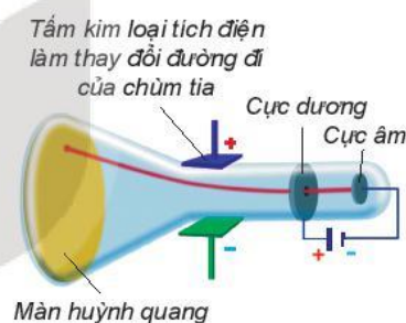
Hình 1.1. Thí nghiệm phát hiện hạt electron
