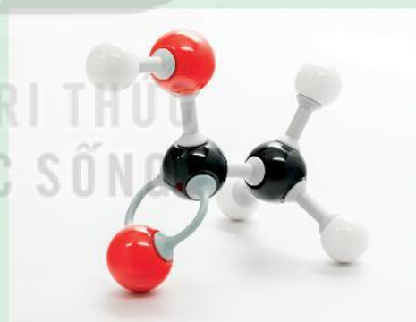
Ethanoic acid ( \text{CH}_3\text{COOH} )
