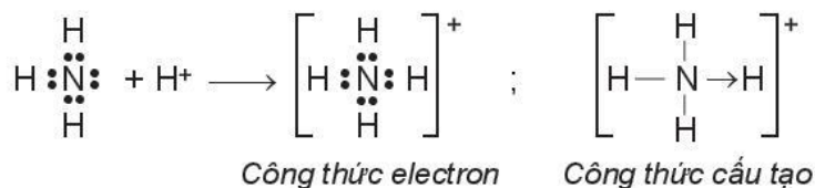
Hình 12.4. Sơ đồ sự tạo thành ion \text{NH}_4^+
