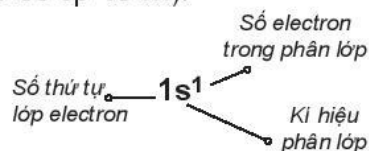
Hình 3.4. Cấu hình electron nguyên tử hydrogen
