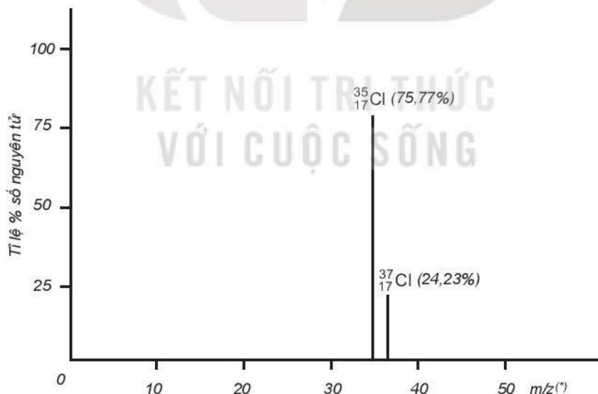
Hình 2.3. Phổ khối lượng của chlorine
