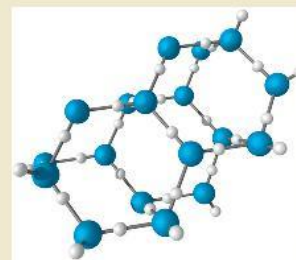
Hình 13.3. Mô hình cấu trúc nước đá
