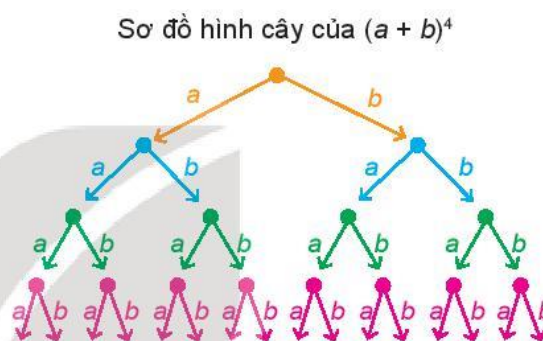
H93. Sơ đồ hình cây của khai triển (a + b)^4 được mô tả như Hình 8.9. Sau khi khai triển, ta thu được một tổng gồm 2^4 (theo quy tắc nhân) đơn thức có dạng x \cdot y \cdot z \cdot t , trong đó mỗi x, y, z, t là a hoặc b . Chẳng hạn, nếu x, y, t là a , còn z là b thì ta có đơn thức a \cdot a \cdot b \cdot a , thu gọn là a^3b . Để có đơn thức này, thì trong 4 nhân tử x, y, z, t có 1 nhân tử là b , 3 nhân tử còn lại là a . Khi đó số đơn thức đồng dạng với a^3b trong tổng là C_4^1 .
