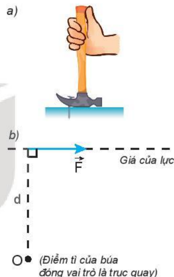
Hình 21.1. Dùng búa nhổ đinh
