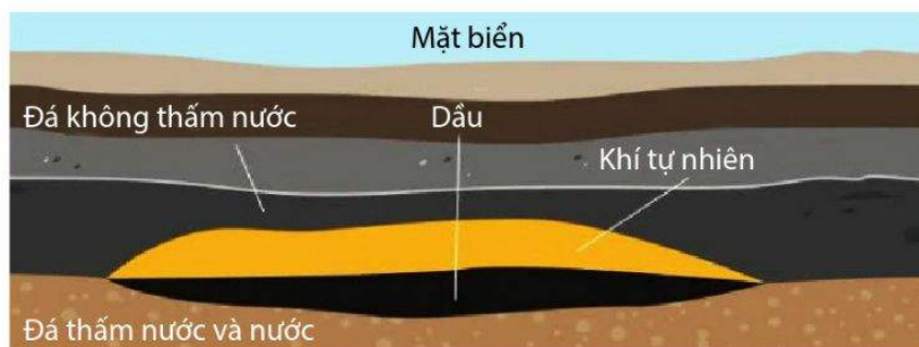
Hình 7.2. Sơ đồ cấu tạo mỏ dầu
