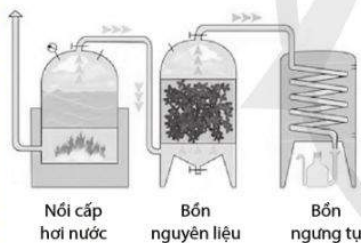
Dụng cụ chưng cất lôi cuốn hơi nước quy mô lớn
