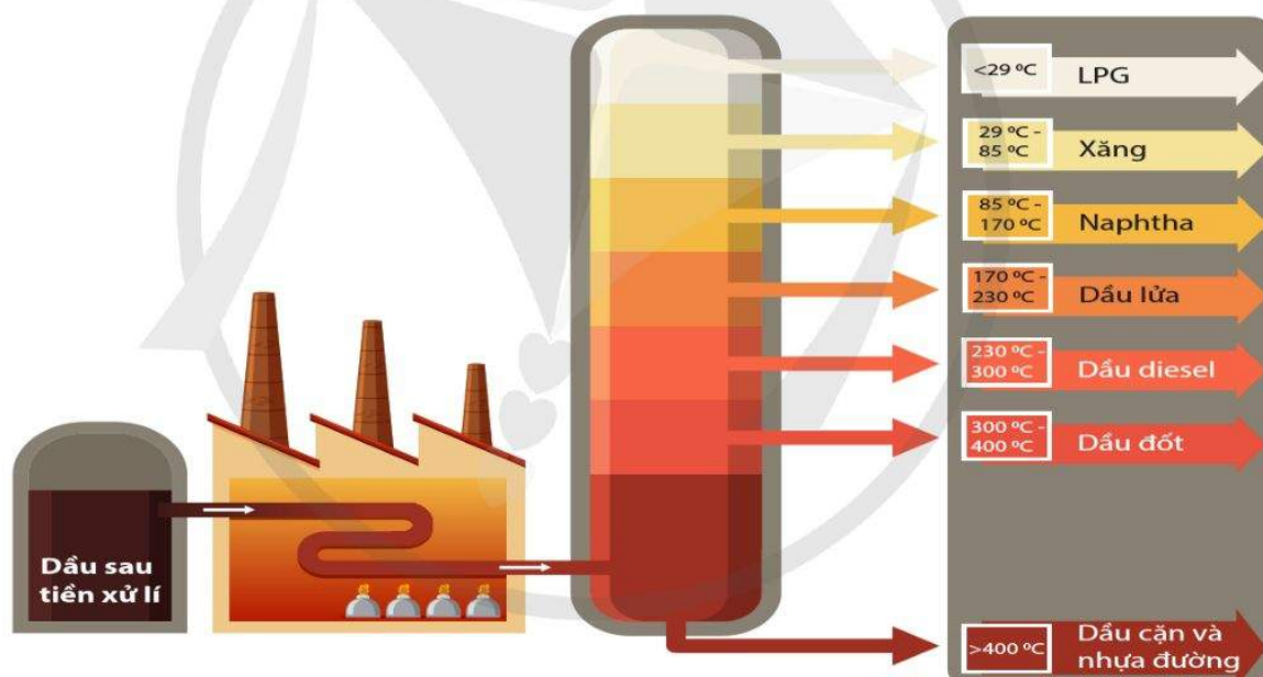
Hình 8.1. Các phân đoạn dầu mỏ từ tháp chưng
