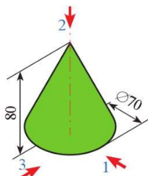
a) Hình nón và các hướng chiếu
