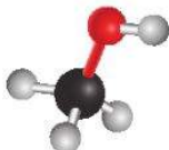
Hình 16.1. Mô hình phân tử methyl alcohol
