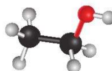
Hình 16.2. Mô hình phân tử ethyl alcohol
