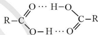
b) Dạng dimer vòng
