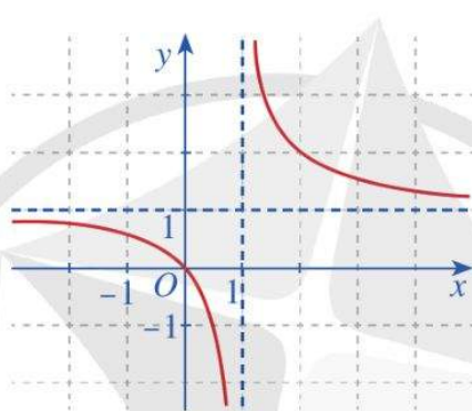
b) Đồ thị hàm số g(x) = \frac{x}{x-1}
