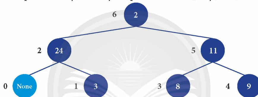
Hình 7. Quá trình duyệt sau cây nhị phân
