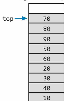
Hình 5a. Ngăn xếp
