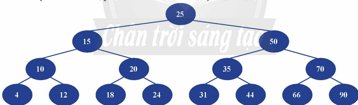
Hình 9. Cây tìm kiếm nhị phân
