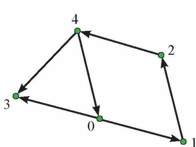
Hình 4. Đồ thị G_4
