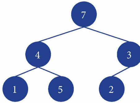
Hình 3. Cây nhị phân
