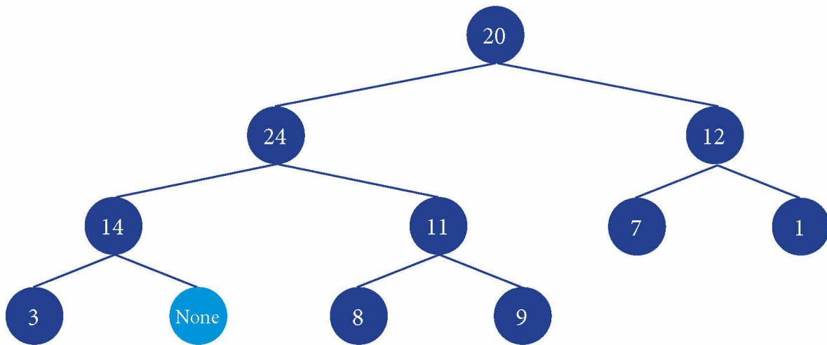
Hình 8. Cây nhị phân
