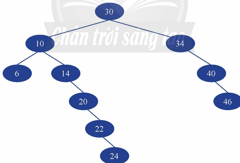
Hình 1. Cây nhị phân
