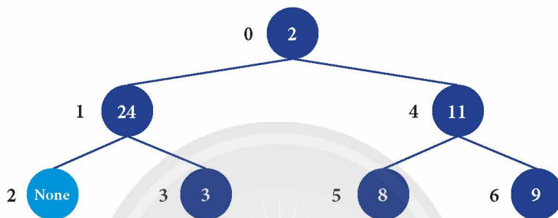
Hình 5. Quá trình duyệt trước cây nhị phân
