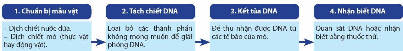
Hình 2.1. Quy trình chung tách chiết DNA từ tế bào
