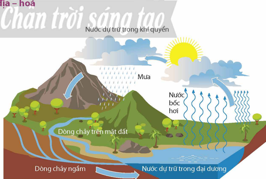
Hình 25.8. Chu trình tuần hoàn nước trong tự nhiên
