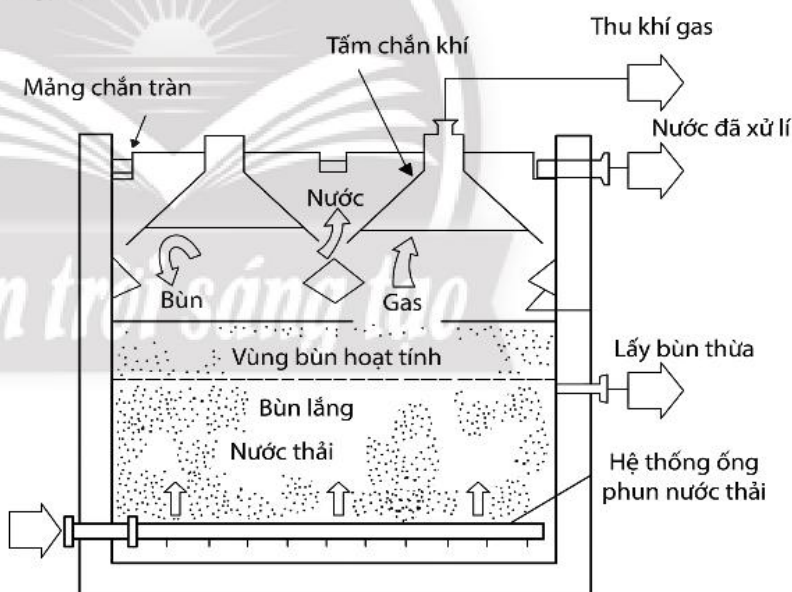
Hình 27.5. Quy trình xử lí nước thải theo phương pháp bùn hoạt tính
