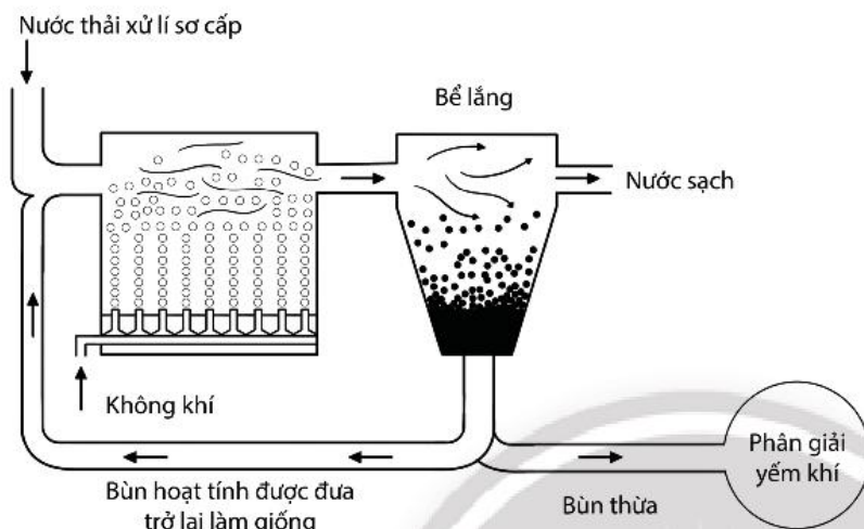
Hình 27.5. Quy trình xử lí nước thải theo phương pháp bùn hoạt tính
