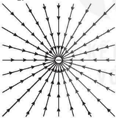
Hình 17.6. Điện phổ của một điện tích âm
