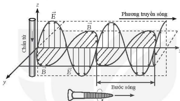
Hình 11.1. Sự lan truyền của sóng điện từ
